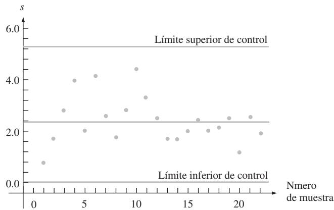
Figura 16.3 Gráfica S para datos de resistencia al esfuerzo del ejemplo 16.4.
