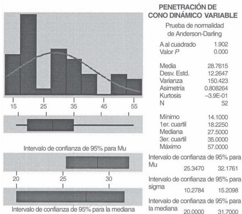
Figura 8.3 Resumen descriptivo generado por MINITAB para los datos de penetración de cono dinámico del ejemplo 8.8.
