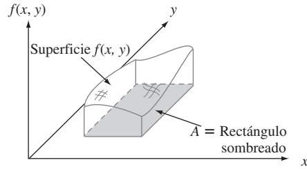
Figura 5.1 P[(X, Y) \in A] = \text{volumen bajo la superficie de densidad sobre } A .
