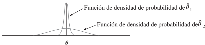
Figura 6.3 Gráficas de las funciones de densidad de probabilidad de dos estimadores inesgados diferentes.
