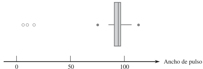
Figura 1.20 Gráfica de caja de los datos de ancho de pulso que muestra valores apartados moderados y extremos.
