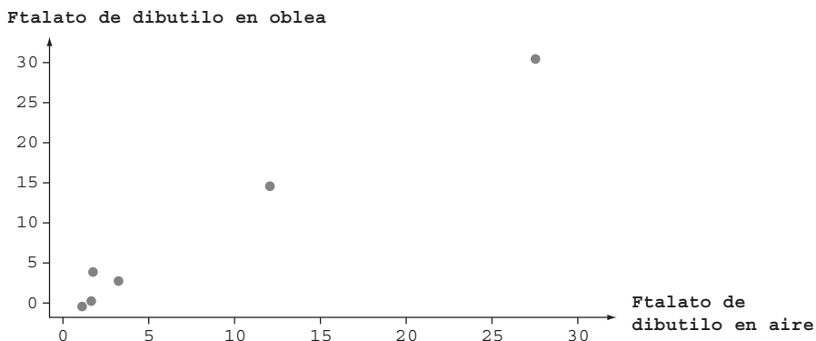
Figura 6.2 Gráfica de los datos de ftalato de dibutilo del ejemplo 6.5.
