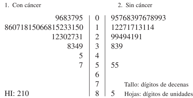
Figura 1.21 Gráfica de tallo y hojas del ejemplo 1.19.
