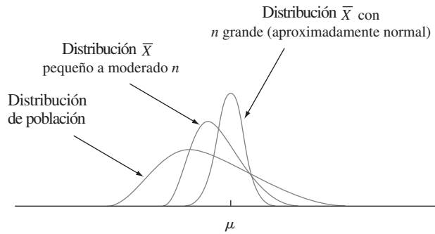
Figura 5.15 Teorema del límite central ilustrado.
