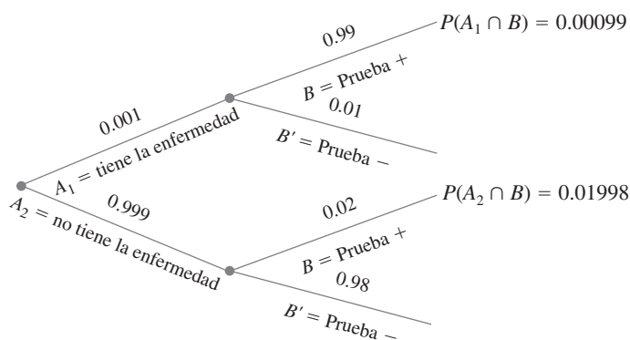
Figura 2.12 Diagrama de árbol para el problema de la enfermedad rara.
