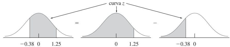
Figura 4.16 P(-0.38 \leq Z \leq 1.25) como la diferencia entre dos áreas acumulativas.
