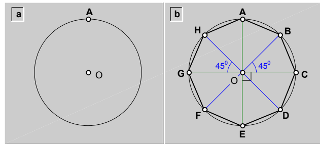
fig.35.1 Dibujo de un octágono regular (ABCDEFGH), conocido el vértice (A) y la circunferencia que lo circunscribe.
