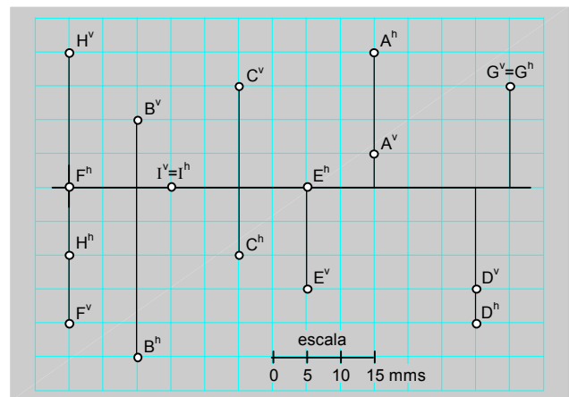
fig.82.1 Proyección de puntos ejemplo.
