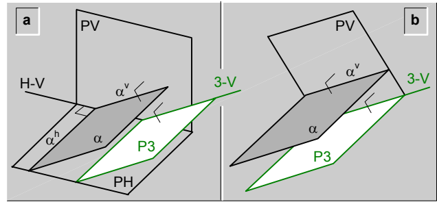
fig.265.1 Cambio del plano horizontal de proyección, para observar en posición horizontal a un plano de punta.
