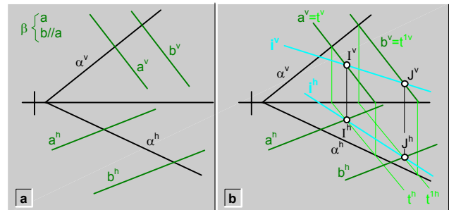
fig.151.\ Intersección (i), entre un plano ( \alpha ) definido por trazas, y un plano ( \beta ) definido por rectas (a y b) paralelas.
