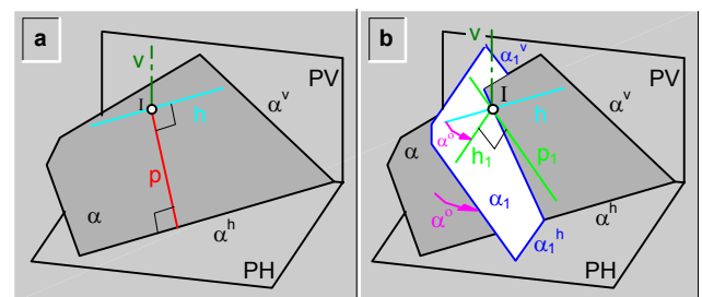
fig.255.\ Rotación de rectas horizontal (h) y de máxima pendiente (p) a posiciones de punta ( h_1 ) y frontal ( p_1 ), respectivamente.
