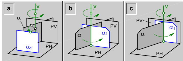
fig.250.\ Rotación de un plano ( \alpha ) en posición vertical a una posición ( \alpha_1 ) frontal.
