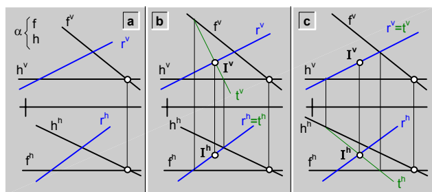
fig.144.\ Intersección (I) de la recta (r) con el plano (α) definido por rectas características (f y h).
