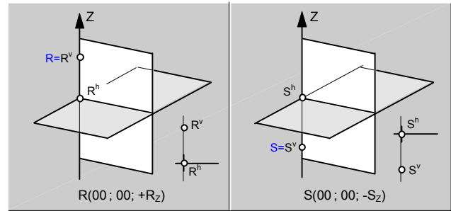
fig.74.\ Punto en el eje (Z).
