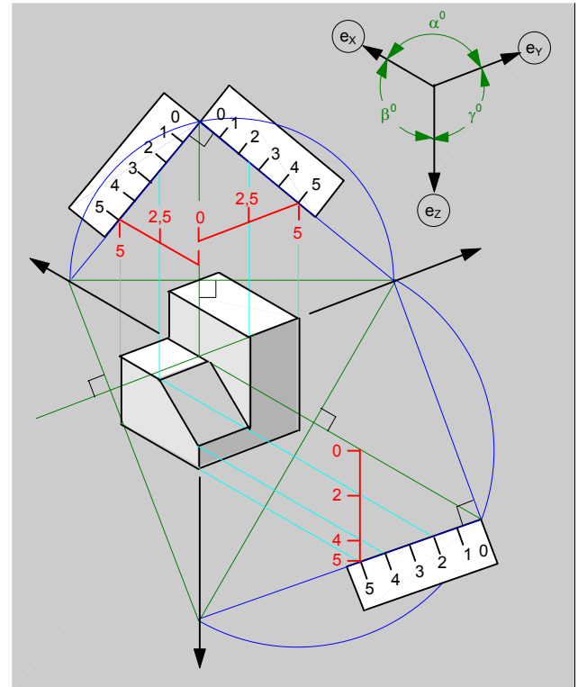
fig.52.\ Proyección trimétrica.
