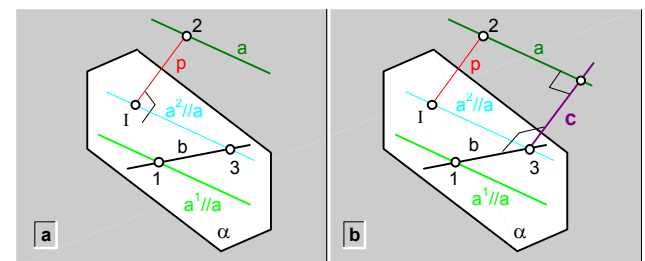
fig.189.\ Perpendicular común (c) a dos rectas (a y b) que se cruzan.
