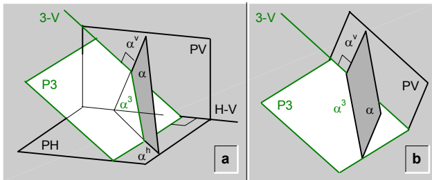
fig.269. Cambio del plano horizontal de proyección, para observar en posición vertical a un plano cualquiera.
