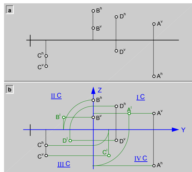
fig.79.1 Obtención de las proyecciones laterales a partir de la doble proyección ortogonal ejemplo.
