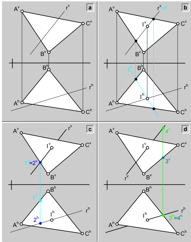
fig.148.\ Intersección entre recta y plano\ VISIBILIDAD.
