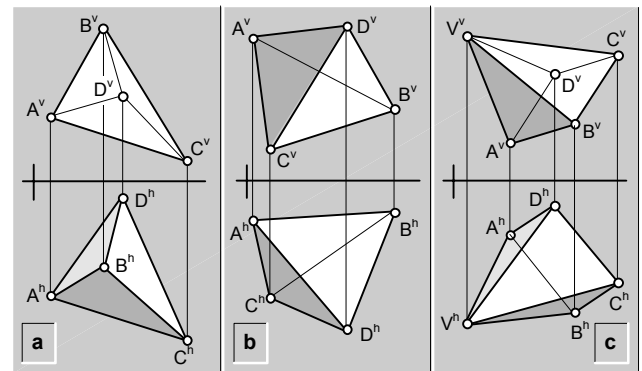
fig.277.\ Visibilidad en poliedros\ ejemplos.
