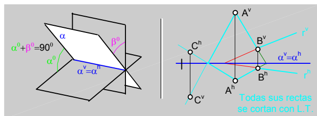
fig.138. Plano que pasa por la línea de tierra.
