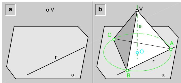
fig.298.\ Construcción de una pirámide regular recta, conocido el vértice principal, y el plano base con una recta que contiene a una arista de la base.
