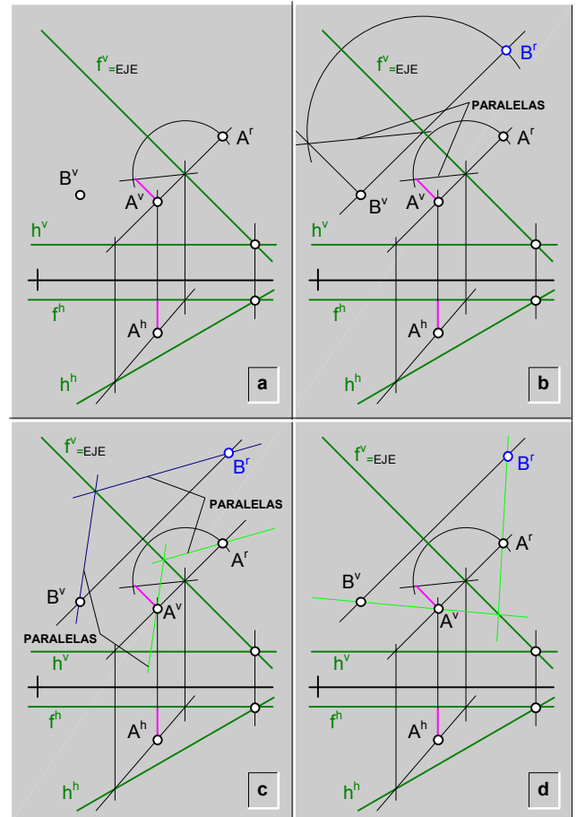
fig.235.\ Rebatimiento de varios puntos.
