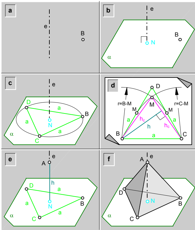
fig.279.\ Construcción de un tetraedro regular, dado un vértice (B) y una recta (e) que contiene a un eje.
