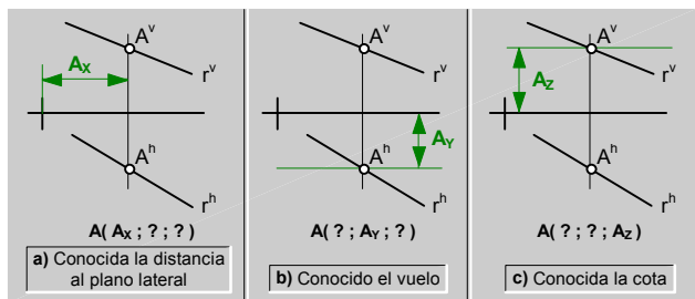
fig.85.\ Ubicación de un punto ( A ) en una recta ( r ).
