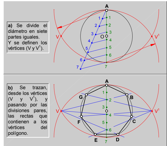
fig.37.1 Dibujo de un heptágono regular, (Método general).
