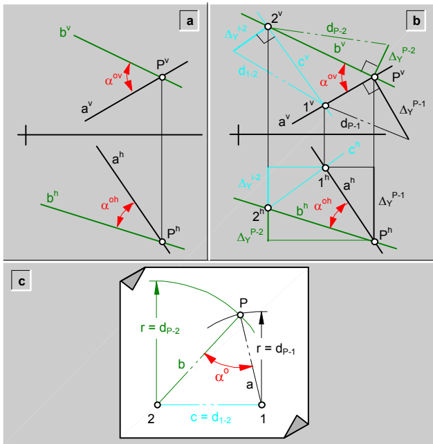
fig.191.\ Ángulo ( \alpha^\circ ) entre dos rectas (a y b) que se cortan.
