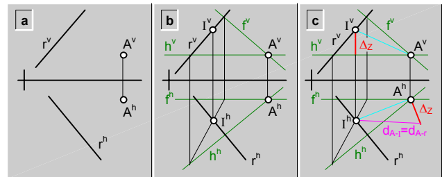
fig.186.\ Distancia ( d_{A-r} ) entre un punto (A) y una recta (r)\ ejemplo.
