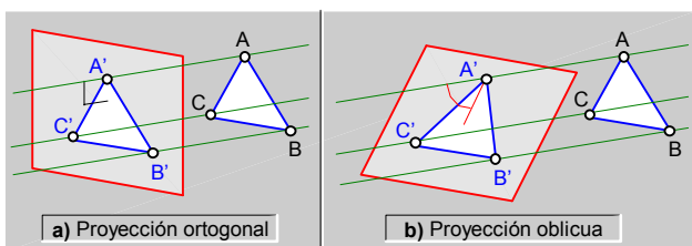
fig.44.\ Proyección cilíndrica.
