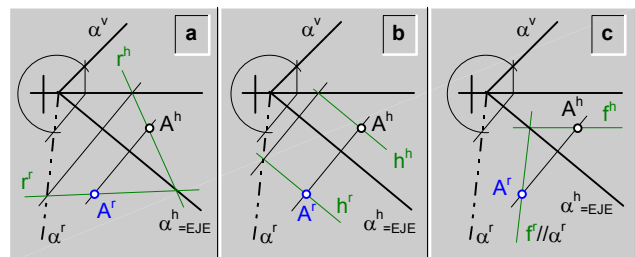
fig.222.1 Rebatimiento de un punto (A), por medio del rebatimiento previo de la traza vertical del plano.
