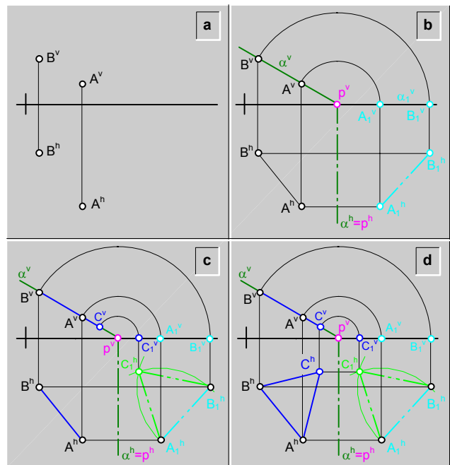
fig.259.\ Rotación de un plano de punta a una posición horizontal.
