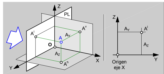
fig.76.\ Proyección lateral.
