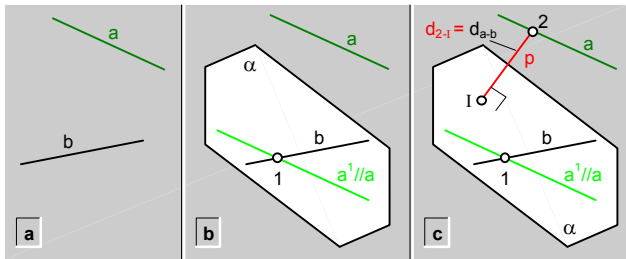
fig.187.\ Distancia ( d_{a-b} ) entre dos rectas (a y b) que se cruzan.
