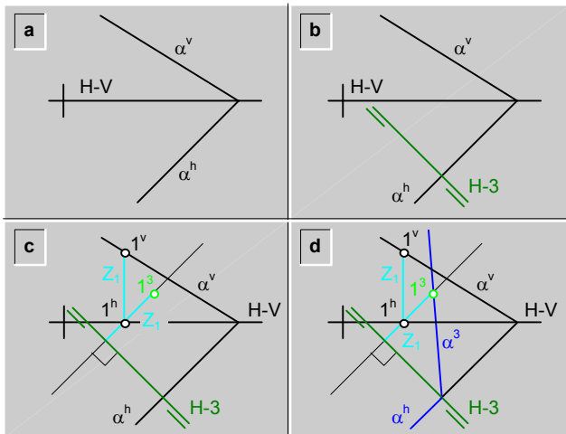
fig.264.1 Cambio del plano vertical de proyección, para observar en posición de punta a un plano cualquiera\ ejemplo.
