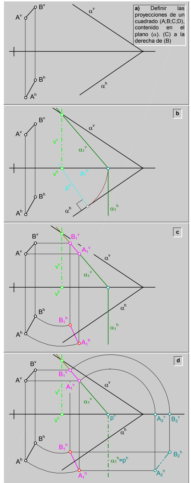
fig.261.\ Rotación de un plano a una posición horizontal\ ejemplo.
