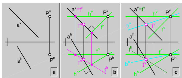
fig.174. Recta ( b ), que contiene a un punto ( P ), y es perpendicular a otra recta ( a )\ ejemplo.
