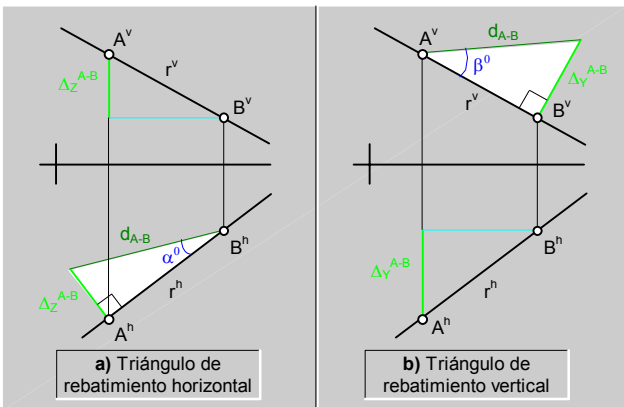
fig.91. \ Dibujo de los triángulos de rebatimiento.
