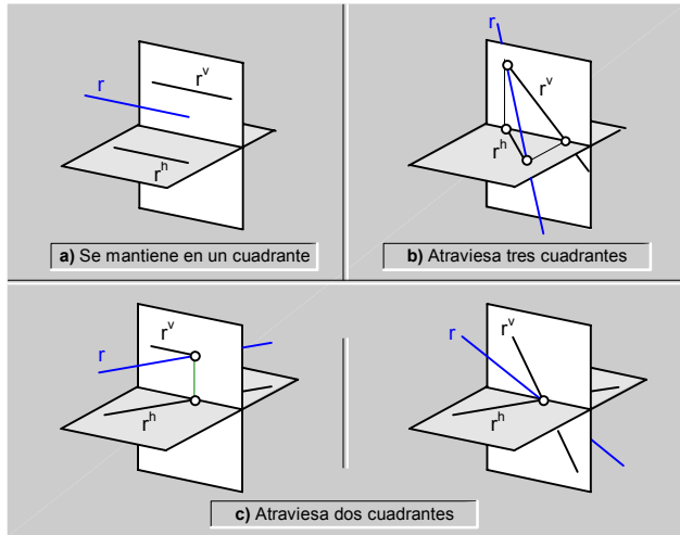
fig.87. \ Recta que atraviesa 1, 2 ó 3 cuadrantes.
