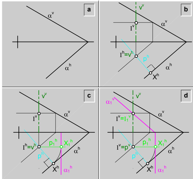
fig.256.\ Rotación de un plano a una posición de punta ejemplo.
