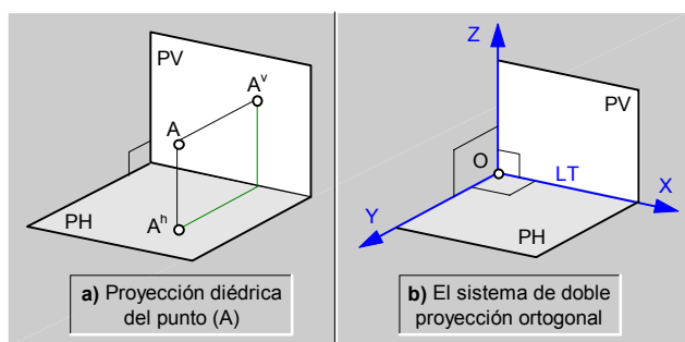
fig.65. La doble proyección ortogonal (proyección diédrica).
