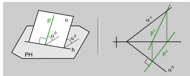
fig.175. Recta ( p ) de máxima pendiente de un plano ( \alpha ).
