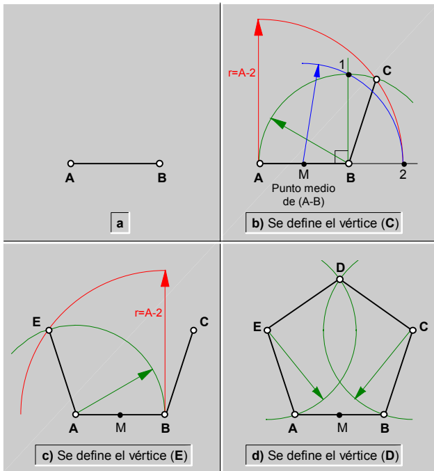
fig.28.\ Dibujo de un pentágono regular (ABCDE), conocido el lado (AB).
