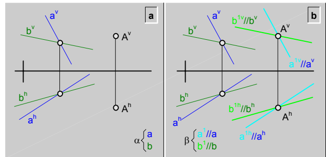
fig.164. Paralelismo entre planos\ ejemplo 1.
