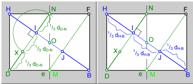
fig.288.\ Propiedades geométricas de toda sección principal de un cubo.
