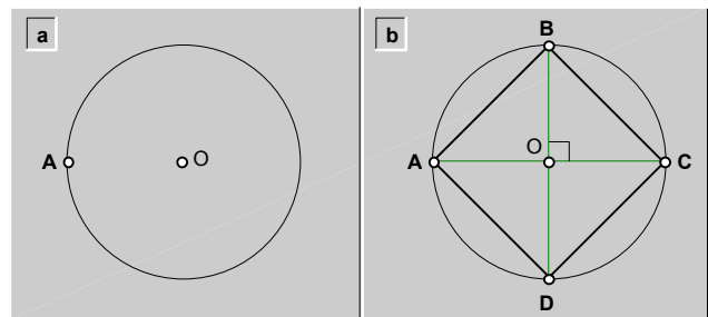
fig.27.\ Dibujo de un cuadrado (ABCD), conocido el vértice (A), y la circunferencia que lo circunscribe.
