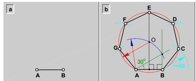
fig.32.\ Dibujo de un heptágono regular (ABCDEFG), conocido el lado (AB).
