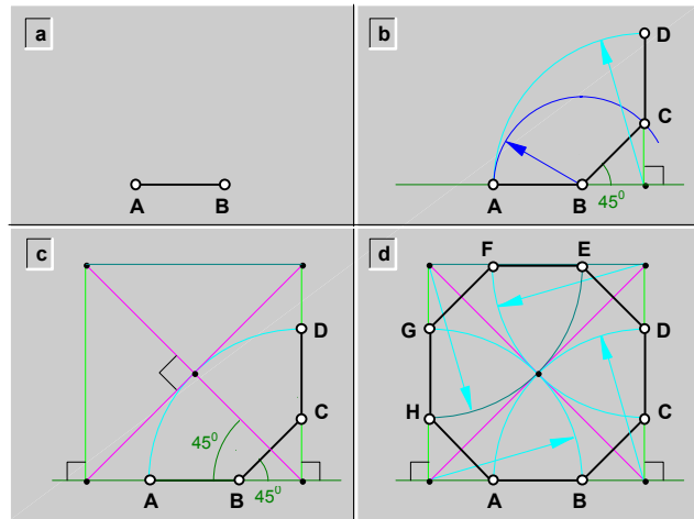
fig.34.1 Dibujo de un octágono regular (ABCDEFGH), conocido el lado (AB).
