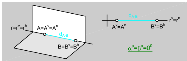
fig.99.\ Recta contenida en la línea de tierra.
