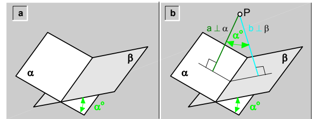
fig.195.\ Ángulo ( \alpha^\circ ) entre dos planos ( \alpha y \beta ).
