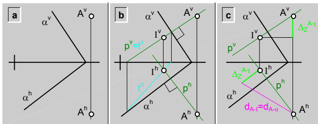
fig.184.\ Distancia ( d_{A-\alpha} ) entre un punto (A) y un plano ( \alpha )\ ejemplo.
