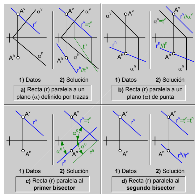
fig.159. Recta (r) paralela a un plano ( \alpha ) ejemplos.
