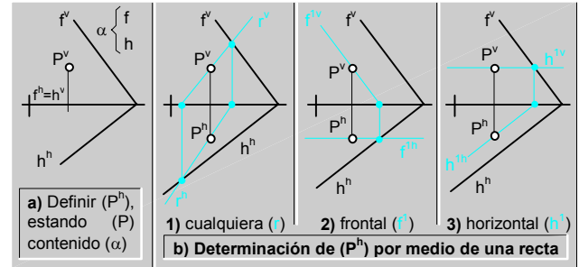
fig.134. \ Punto contenido en un plano definido por trazas.
