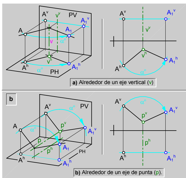
fig.242.\ Rotación de un punto (A) hasta la posición ( A_1 ).
