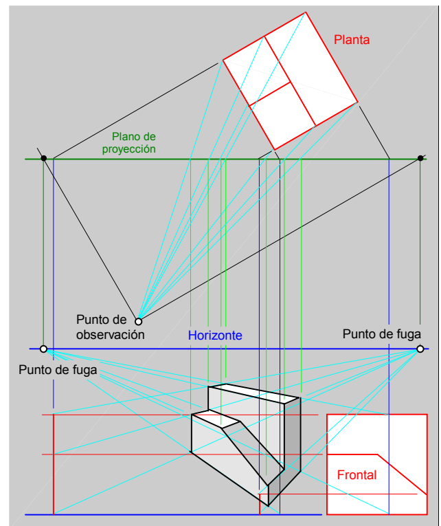
fig.63.\ Dibujo de una perspectiva de dos puntos de fuga.
