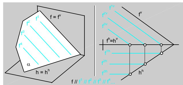
fig.130. Paralelismo entre rectas características frontales.
