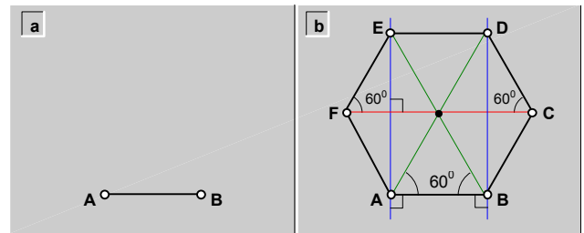
fig.30.\ Dibujo de un hexágono regular (ABCDEF), conocido el lado (AB).
