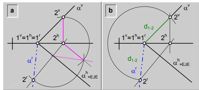
fig.221.1 Rebatimiento de la traza vertical de un plano.
