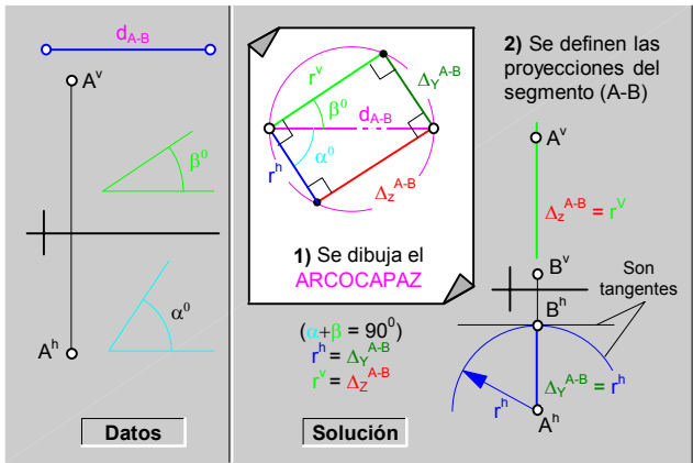
fig.114.\ Construcción de rectas (VT + \alpha^0 + \beta^0 ) \ La solución es una recta de perfil.
