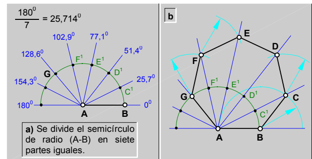
fig.38.1 Dibujo de un heptágono regular, (Método general).
