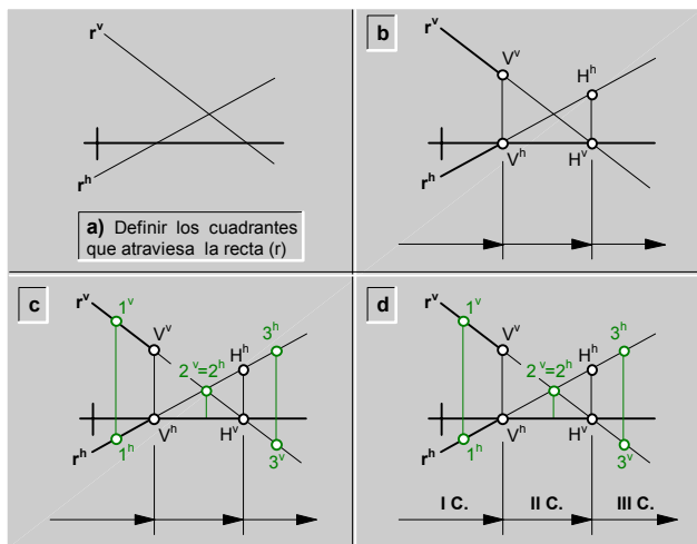
fig.88. \ Determinación de los cuadrantes que atraviesa una recta.
