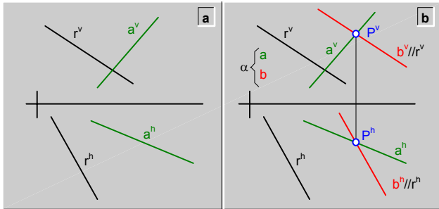
fig.160. Plano ( \alpha ), paralelo a una recta ( r )\ ejemplo.
