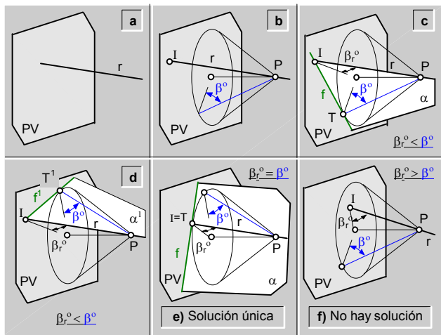
fig.209.\ Plano ( \alpha ) que contiene a una recta ( r ) dada y forma un ángulo ( \beta^\circ ) dado con el plano vertical de proyección.
