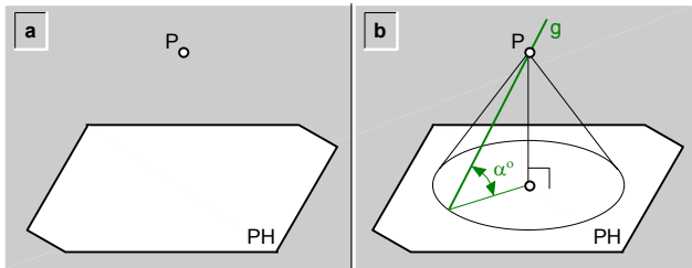
fig.203.\ Recta ( g ) que contiene a un punto ( P ) dado y forma un ángulo ( \alpha^\circ ) dado con el plano horizontal de proyección.
