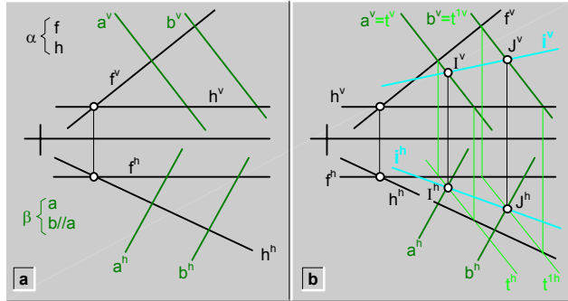
fig.152.\ Intersección (i), entre un plano ( \alpha ) definido por rectas (f y h) características, y un plano ( \beta ) definido por rectas (a y b) paralelas.
