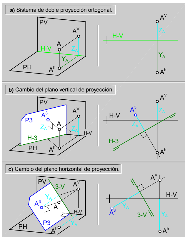
fig.262.\ Cambio de planos de proyección.
