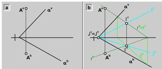
fig.153.\ Intersección (i) de un plano ( \alpha ) definido por trazas, con un plano ( \beta ) que pasa por la línea de tierra y contiene a un punto (A).
