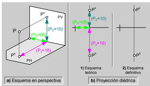
fig.68.\ Representación diédrica del punto P(08 ; 16 ; 10).
