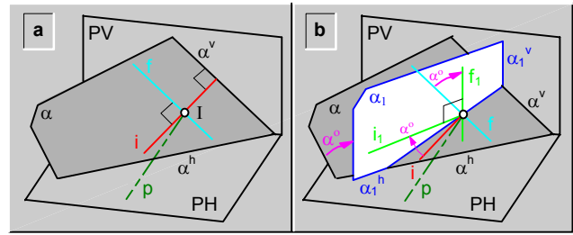
fig.247.\ Rotación de rectas frontal (f) y de máxima inclinación (i) a posiciones vertical ( f_1 ) y horizontal ( i_1 ), respectivamente.
