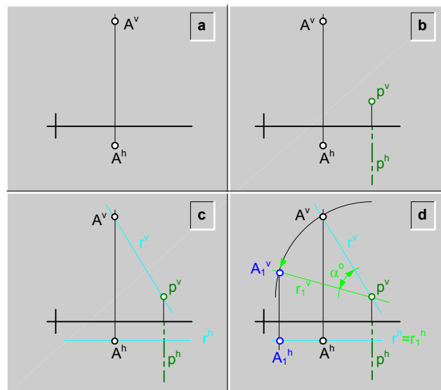
fig.243.\ Rotación alrededor de un eje de punta.
