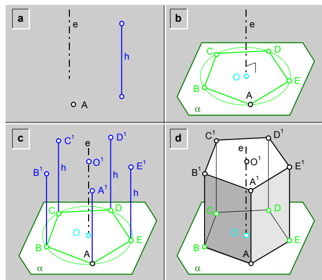
fig.303.\ Construcción de un prisma regular recto, conocido: la altura; un vértice; y la recta ( e ) que contiene al eje.
