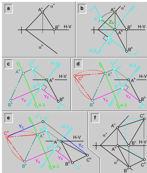
fig.268.\ Observación en posición horizontal de un plano cualquiera, por medio de dos cambios de plano de proyección ejemplo.
