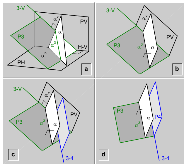
fig.273.\ Observación de un plano en posición frontal por medio de dos cambios de plano.
