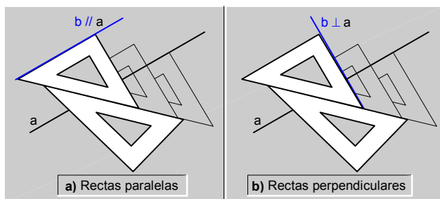
fig.17.\ Trazado de rectas paralelas; y perpendiculares.
