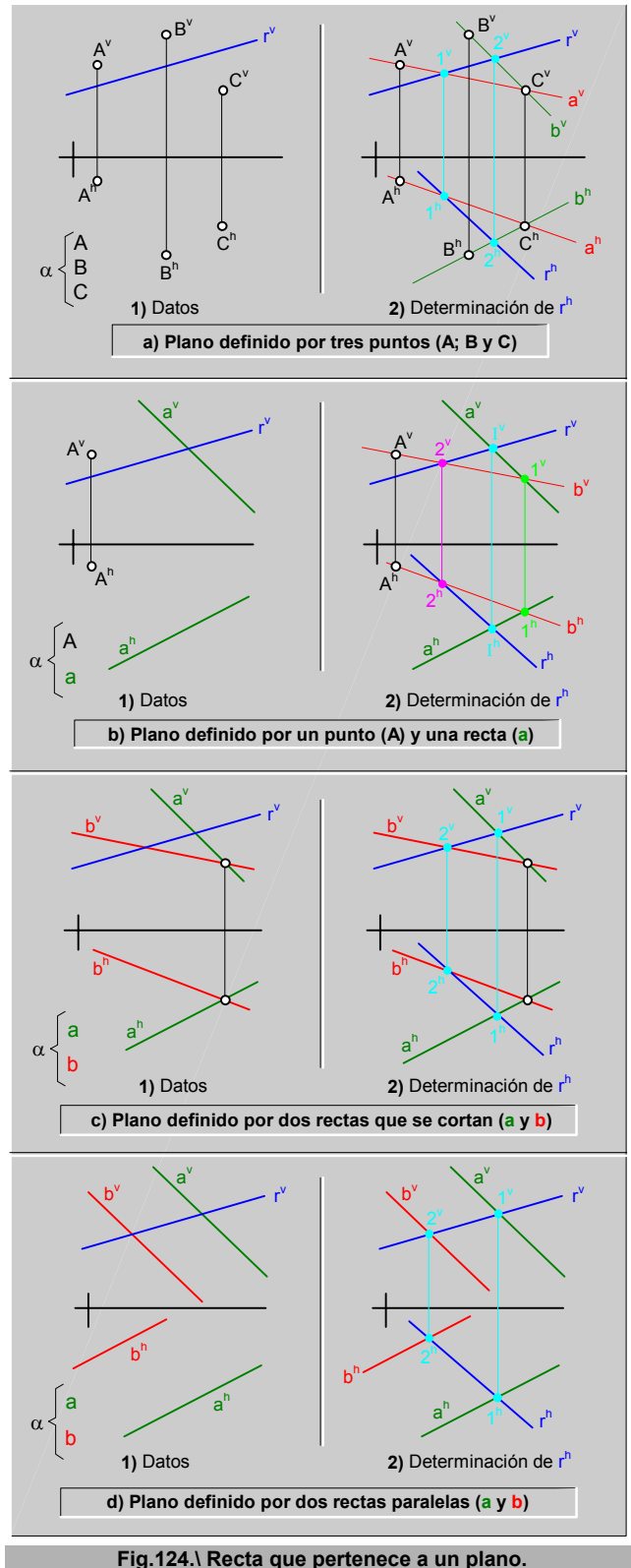
Fig.124. Recta que pertenece a un plano.
