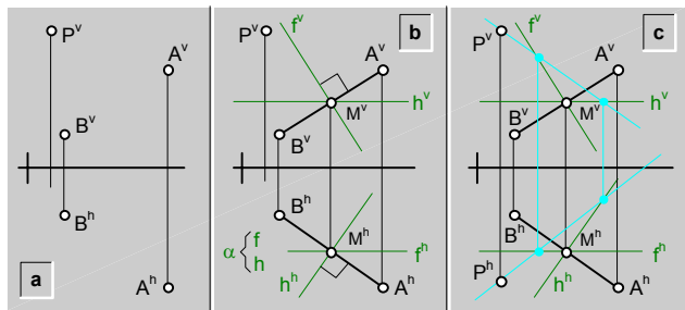
fig.198.\ Punto (P) que equidista de dos puntos (A y B) dados \ ejemplo.
