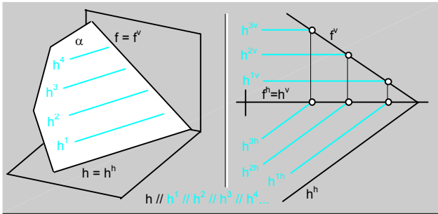
fig.131. \ Paralelismo entre rectas características horizontales.
