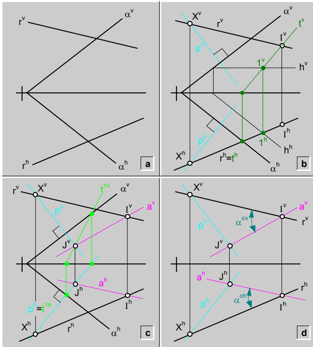
fig.194.\ Ángulo ( \alpha^\circ ) entre una recta (r) y un plano ( \alpha )\ ejemplo.
