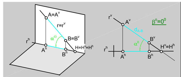
fig.97.\ Recta contenida en el plano vertical de proyección.
