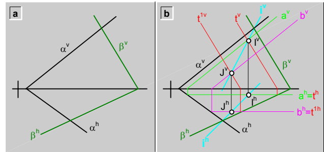
fig.150.\ Intersección (i), entre dos planos ( \alpha y \beta ) definidos por trazas.
