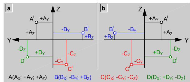
fig.77.1 Proyección lateral ejemplos.
