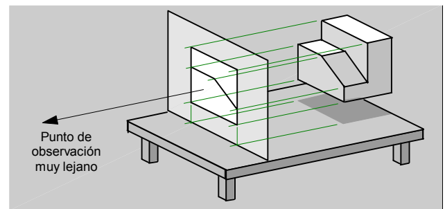
fig.45.\ Vista ortográfica.
