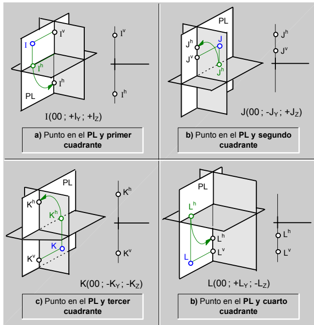
fig.71.\ Ubicación de un punto en el plano lateral.
