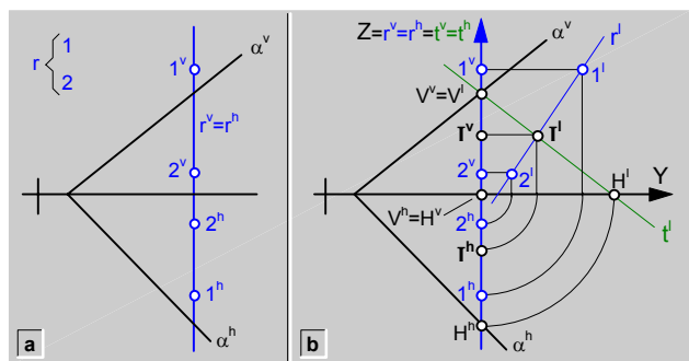
fig.145.\ Intersección (I) de un plano (α) definido por trazas, con una recta (r) de perfil.
