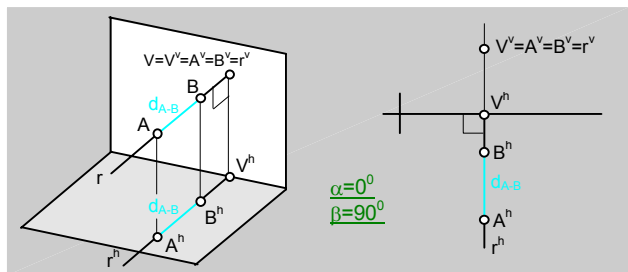
fig.101.\ Recta de punta.
