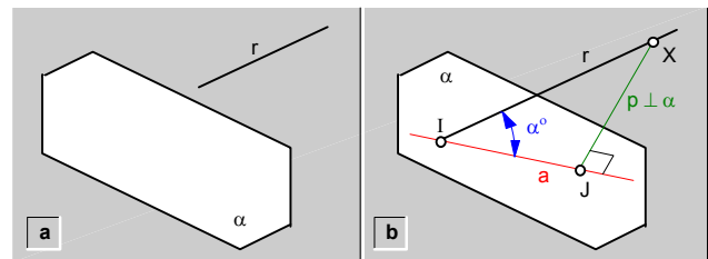
fig.193.\ Ángulo ( \alpha^\circ ) entre una recta (r) y un plano ( \alpha ).
