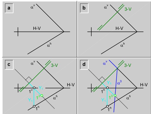
fig.270. Cambio del plano horizontal de proyección, para observar en posición vertical a un plano cualquiera ejemplo.
