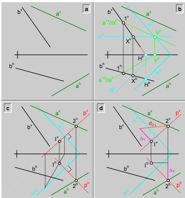
fig.188.\ Distancia ( d_{a-b} ) entre dos rectas (a y b) que se cruzan\ ejemplo.
