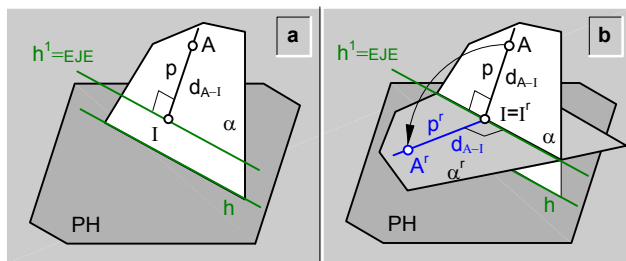
fig.228.\ Rebatimiento a través de una recta característica horizontal ( h^1 ) del plano ( \alpha ).
