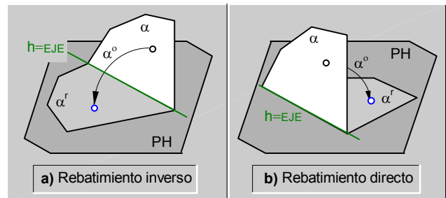
fig.217.\ Rebatimiento inverso y rebatimiento directo.
