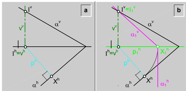
fig.257.\ Eje de rotación en el plano vertical de proyección.
