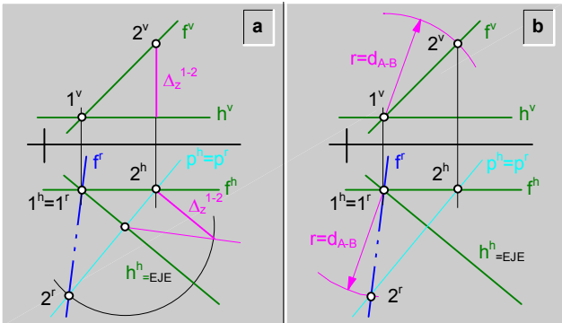
fig.231.1 Rebatimiento de una frontal de un plano ( \alpha ).
