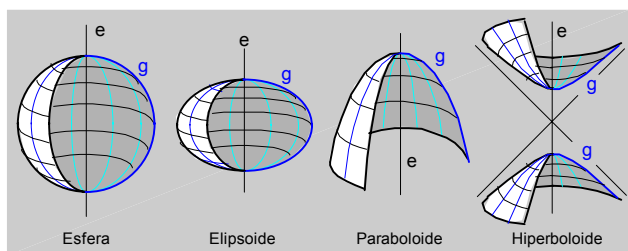
fig.12.\ Superficies de doble curvatura.
