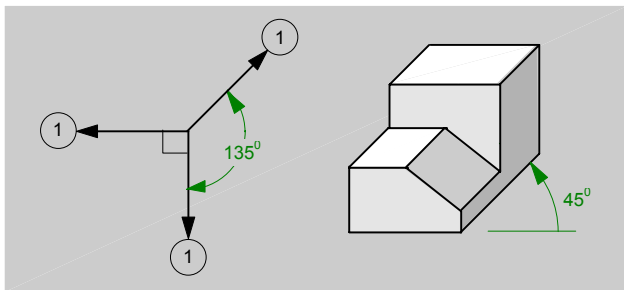
fig.55.\ Proyección caballera.
