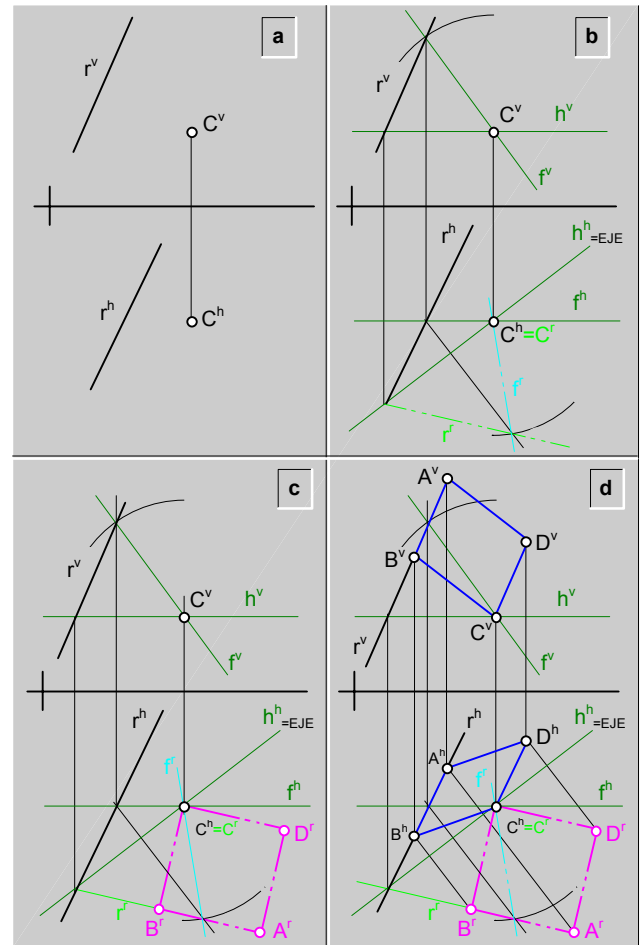
fig.240. \ Construcción de un cuadrado por rebatimiento previo de una recta frontal.
