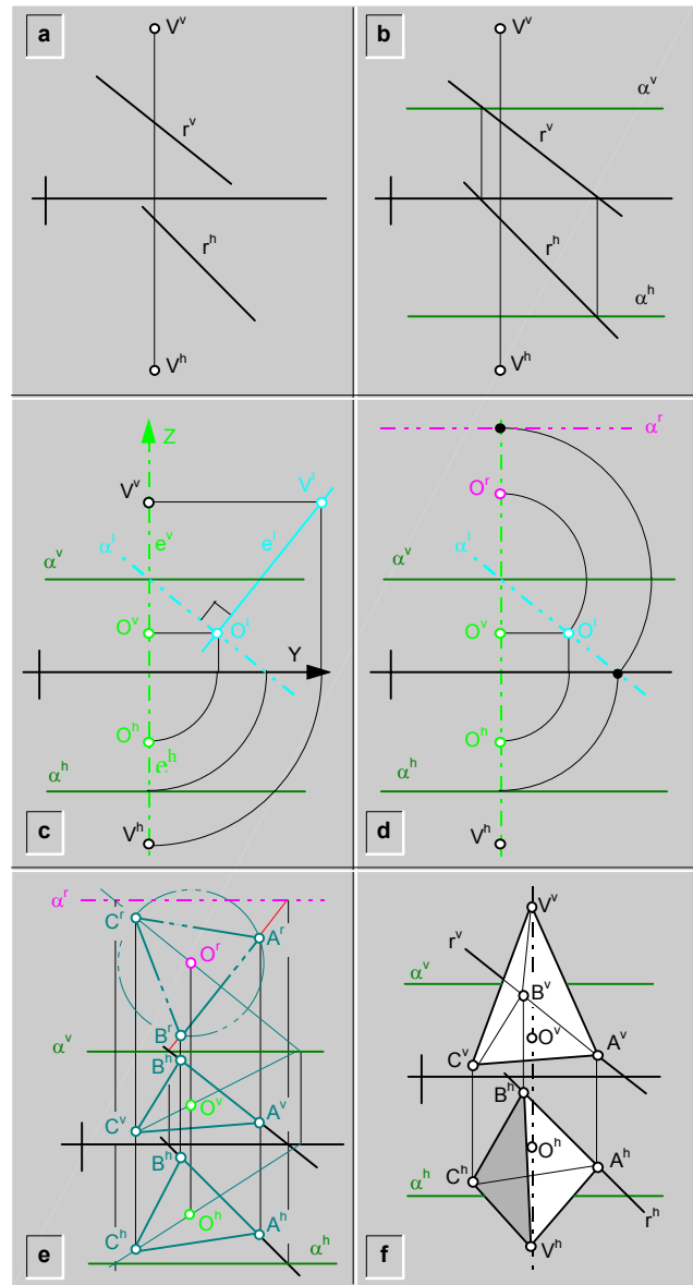
fig.299.\ Construcción de una pirámide regular recta de base triangular (ABC), con vértice principal (V), y plano base ( \alpha ) paralelo a la línea de tierra, dada la recta (r), que contiene a la arista (A-B) de la base\ ejemplo.
