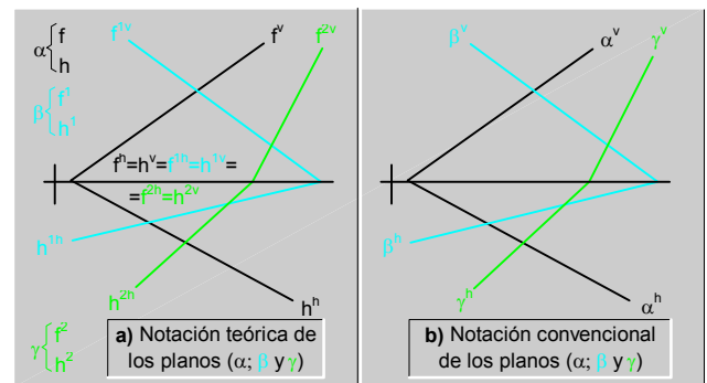
fig.136. \ Notación teórica y convencional de los planos ( \alpha ; \beta y \gamma ).
