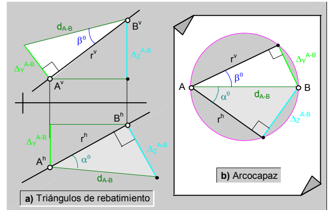
fig.92. \ Arcocapaz.
