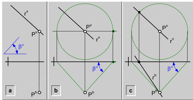
fig.206.\ Recta (r) que contiene a un punto (P) dado y forma un ángulo ( \beta^\circ ) dado con el plano vertical de proyección\ ejemplo.
