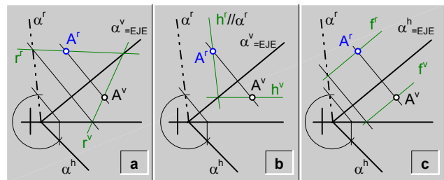
fig.227.1 Rebatimiento de un punto (A) por medio del rebatimiento previo de la traza horizontal del plano.
