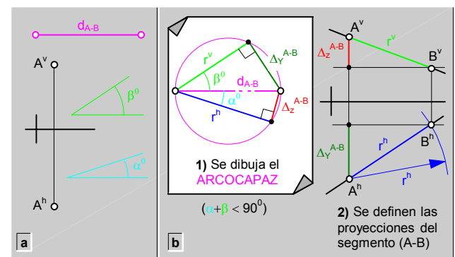
fig.113. Construcción de rectas (VT + \alpha^0 + \beta^0 ).
