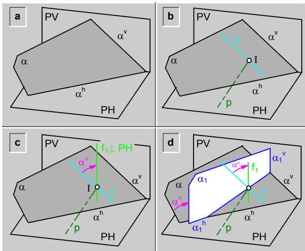
fig.246.\ Rotación de un plano ( \alpha ) a una posición vertical ( \alpha_1 ).
