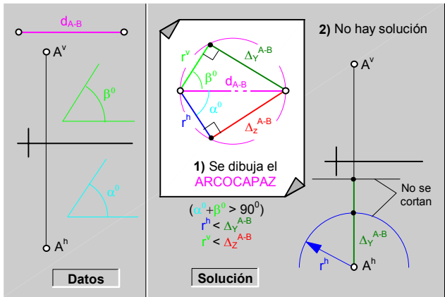
fig.115.\ Construcción de rectas (VT + \alpha^0 + \beta^0 ) \ No hay solución.
