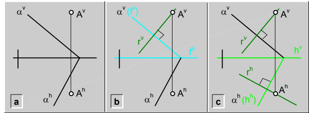
fig.170. \ Recta (r), que contiene a un punto (A) y es perpendicular a un plano ( \alpha ), definido por trazas.
