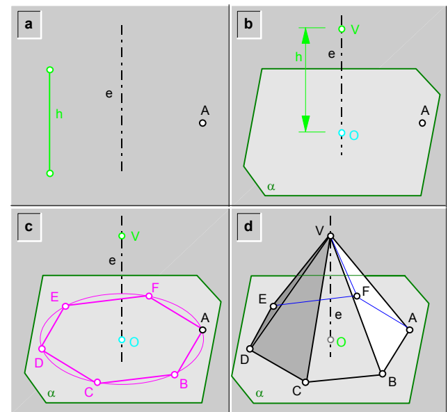
fig.294.\ Construcción de una pirámide regular recta, conocido: la altura (h); un vértice (A) de la base y la recta (e) que contiene al eje.
