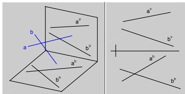
Fig.121.\ Dos rectas (a y b) que se cruzan no definen un plano.
