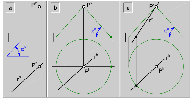
fig.204.\ Recta ( r ) que contiene a un punto ( P ) dado y forma un ángulo ( \alpha^\circ ) dado con el plano horizontal de proyección\ ejemplo.
