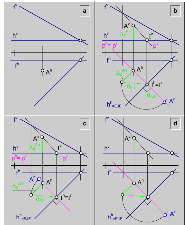
fig.229.\ Rebatimiento alrededor de una recta característica horizontal (h) de un plano ( \alpha ) ejemplo.
