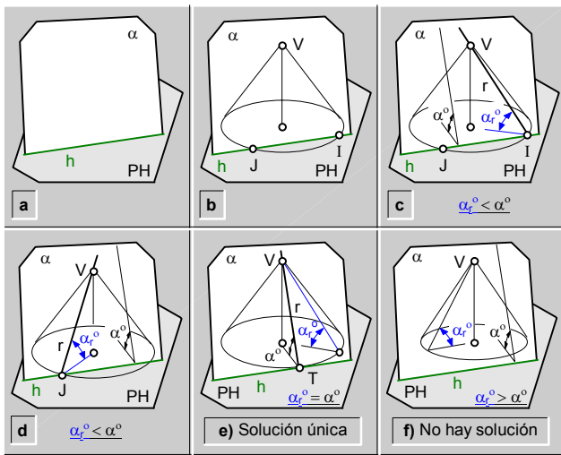
fig.211.\ Recta (r) contenida en un plano ( \alpha ) dado y que forma un ángulo ( \alpha_r^\circ ) dado con el plano horizontal de proyección.
