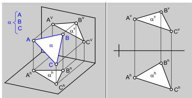
Fig.117.\ Plano ( \alpha ) definido por tres puntos (A; B; y C).
