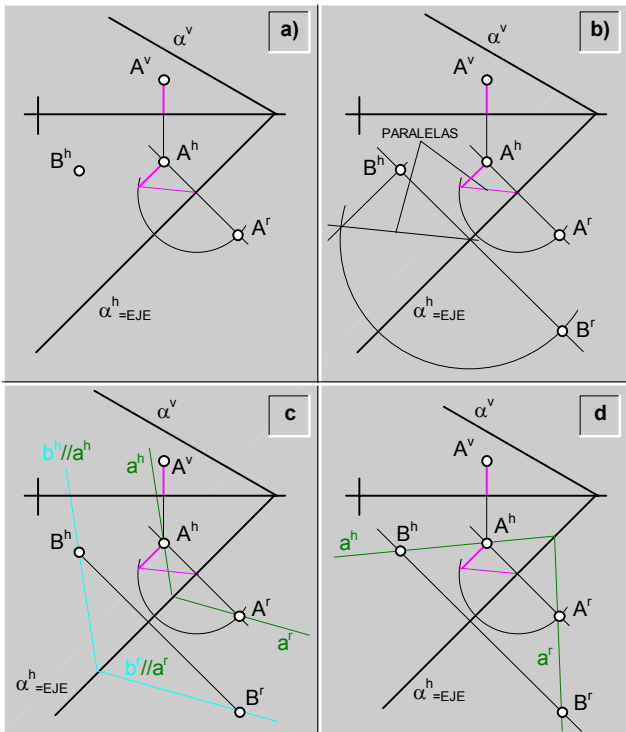
fig.220.1 Rebatimiento de varios puntos.
