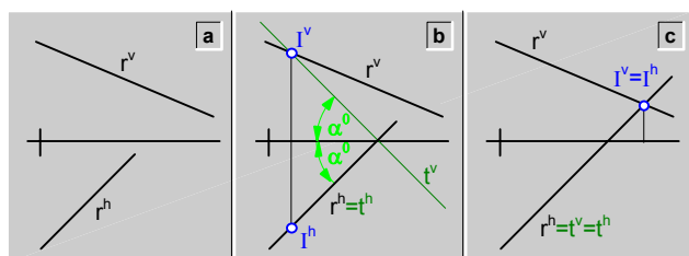
fig.146.\ Intersección (I) de una recta (r) con los planos bisectores.
