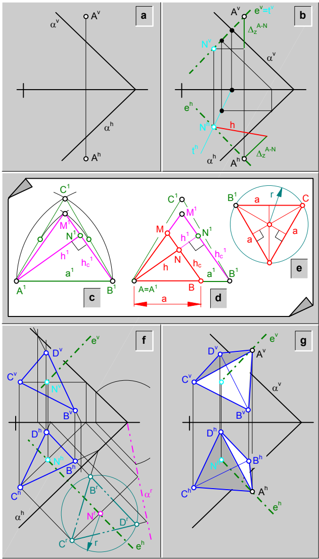
fig.284.\ Construcción de un tetraedro regular, conocido el plano que contiene a una cara y el vértice no contenido en este plano\ ejemplo.
