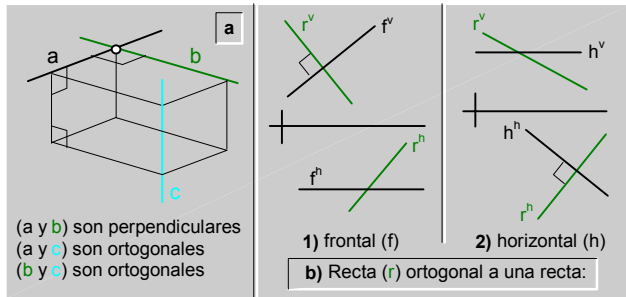
fig.168. \ Perpendicularidad y ortogonalidad.
