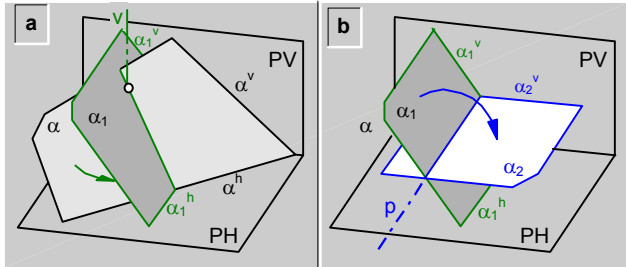
fig.260.\ Rotación de un plano a una posición horizontal.
