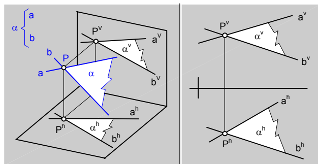
Fig.119.\ Plano ( \alpha ) definido por dos rectas (a y b) que se cortan.
