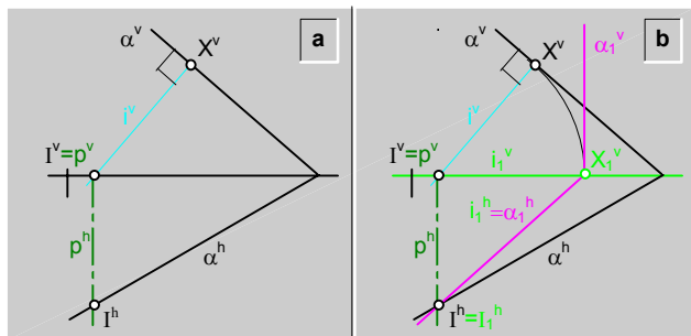
fig.249.\ Eje de rotación en el plano horizontal de proyección .
