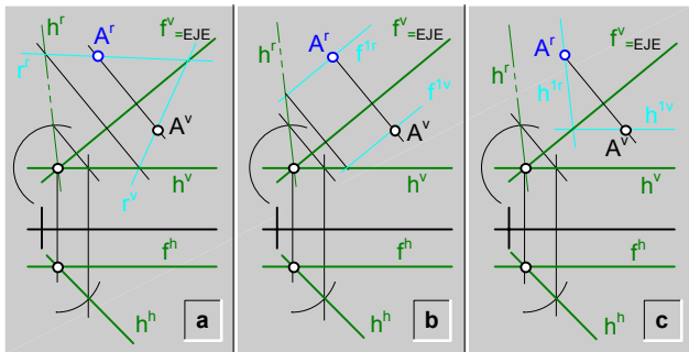
fig.237. \ Rebatiendo de un punto ( A ) de un plano ( \alpha ) por medio del rebatimiento previo de una recta horizontal ( h ).
