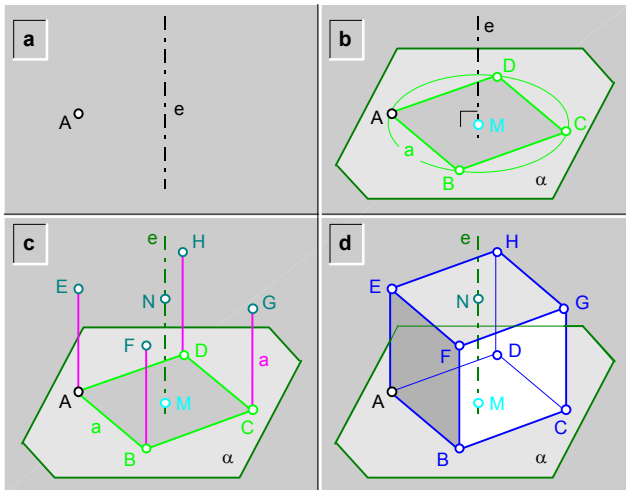
fig.289.\ Construcción de un cubo, conocido un vértice y una recta que contiene a un eje.
