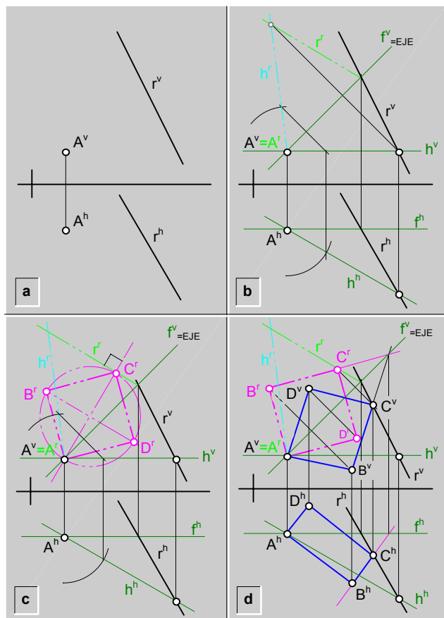
fig.241.\ Construcción de un cuadrado por rebatimiento previo de una recta horizontal.
