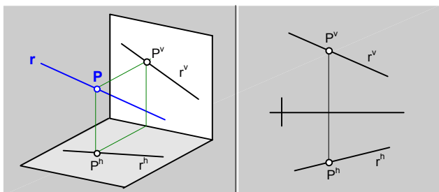
fig.84.\ Punto contenido en una recta.
