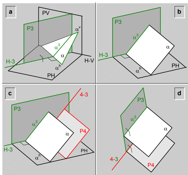
fig.267.\ Observación en posición horizontal de un plano cualquiera, por medio de dos cambios de plano.
