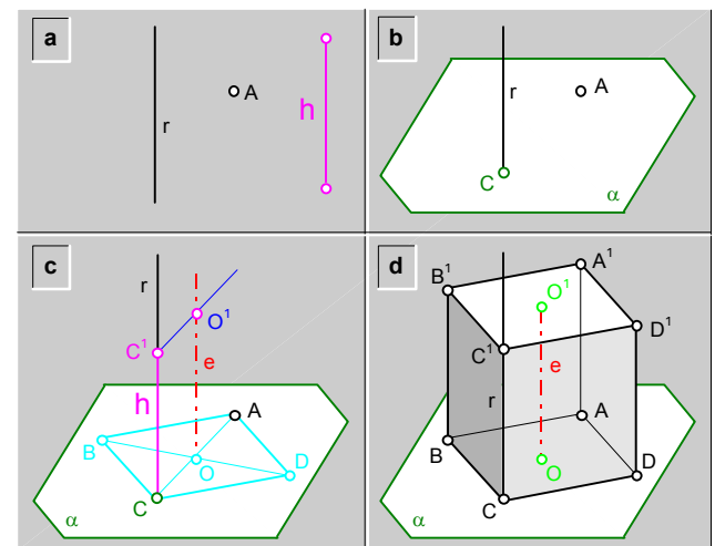
fig.305.1 Construcción de un prisma regular recto, conocida su altura, un vértice y una recta que contiene a una arista principal.
