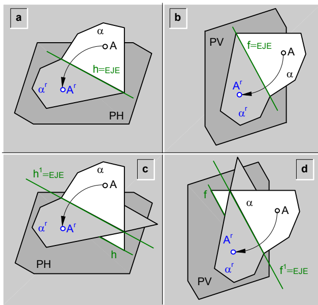
fig.215.\ Rebatimiento de un plano ( \alpha ).
