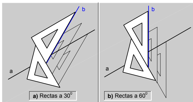
fig.18.\ Trazado de rectas a 30^\circ ; y 60^\circ .
