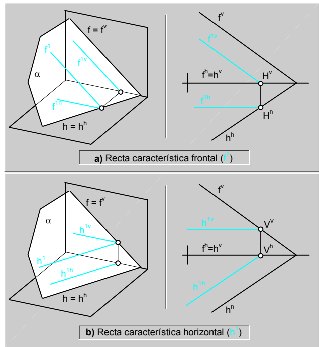
fig.129. Rectas características de un plano.
