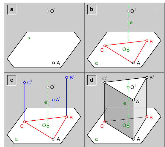
fig.301.\ Construcción de un prisma regular recto, conocido un plano base, con uno de los vértices de la misma, y el centro de la otra base.
