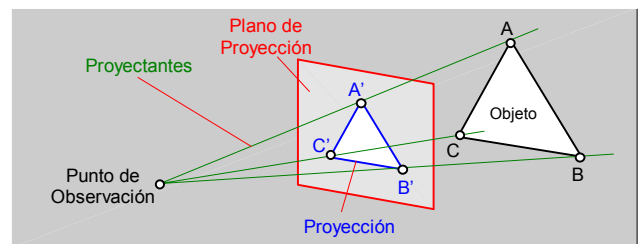
fig.58.\ Proyección cónica.
