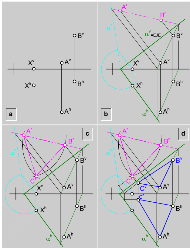
fig.239. \ Construcción de un triángulo equilátero, por rebatimiento previo de la traza horizontal.
