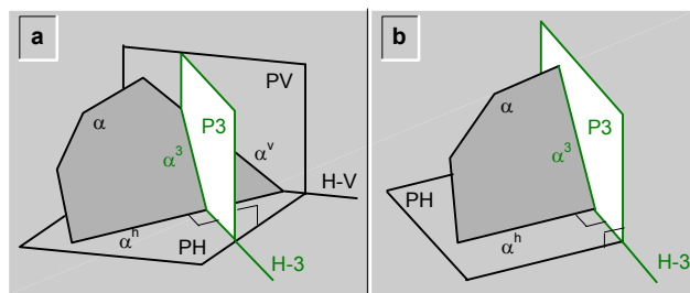
fig.263.\ Cambio del plano vertical de proyección, para observar en posición de punta a un plano cualquiera.
