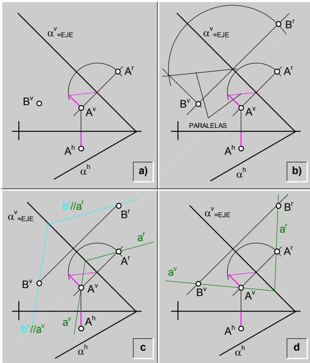
fig.225.1 Rebatimiento de varios puntos.
