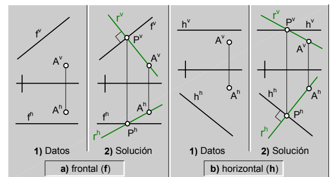
fig.167. Definir las proyecciones de la recta (r) que contiene al punto (A) y es perpendicular a la recta...
