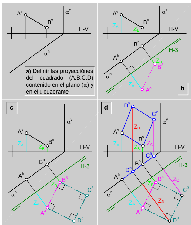
fig.272.\ Cambio del plano vertical de proyección para observar en posición frontal a un plano vertical ejemplo.
