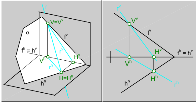
fig.127. Trazas de una recta ( r ) contenida en un plano ( \alpha ).
