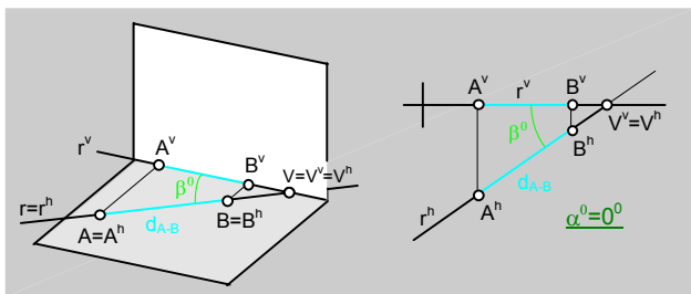
fig.95.\ Recta contenida en el plano horizontal de proyección.
