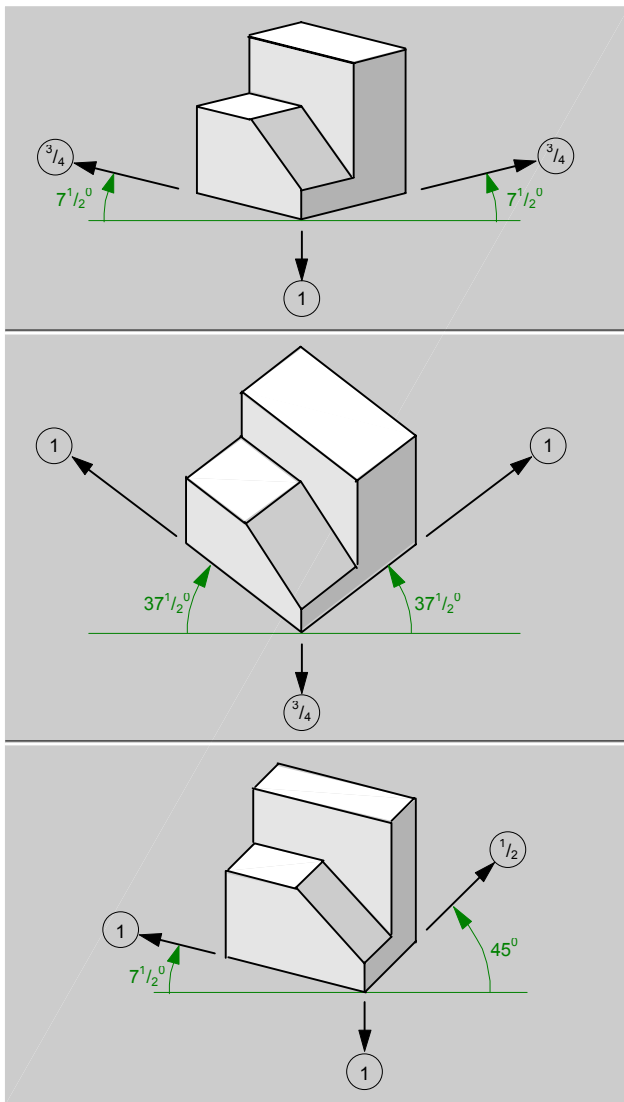
fig.51.\ Proyecciones dimétricas.
