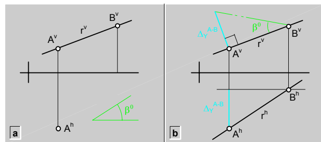
fig.103.\ Construcción de rectas (PV + \beta^0 ).
