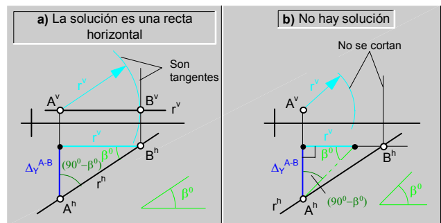
fig.108.\ Construcción de rectas (PH + β) \ casos particulares.
