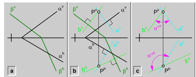
fig.196.\ Ángulo ( \alpha^\circ ) entre dos planos ( \alpha y \beta )\ ejemplo.
