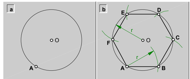
fig.31.\ Dibujo de un hexágono regular (ABCDEF), conocido el vértice (A) y la circunferencia que lo circunscribe.
