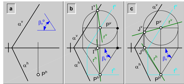
fig.214.\ Recta ( r ) contenida en un plano ( \alpha ) dado y que forma un ángulo ( \beta_r^\circ ) dado con el plano vertical de proyección\ ejemplo.
