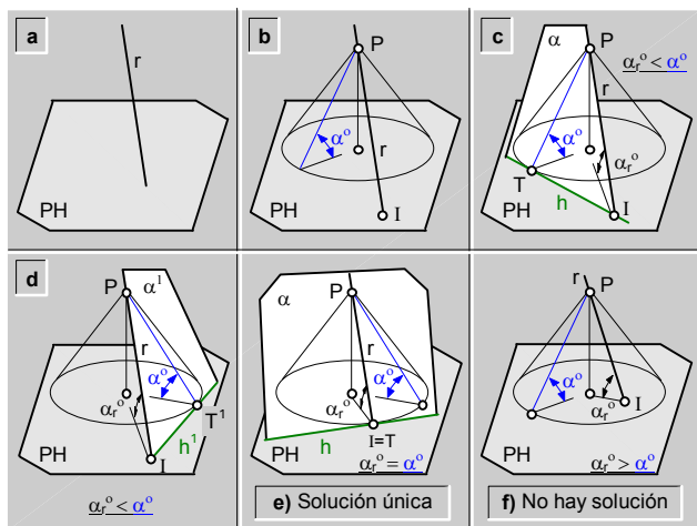
fig.207.\ Plano ( \alpha ) que contiene a una recta (r) dada y forma un ángulo ( \alpha^\circ ) dado con el plano horizontal de proyección.
