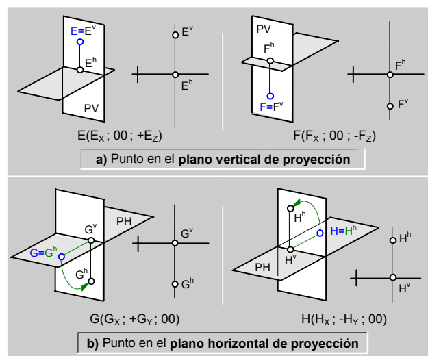
fig.70.\ Ubicación de un punto en un plano principal de proyección.
