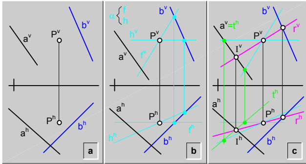
fig.202.\ Recta ( r ) que se corta con dos rectas ( a y b ) dadas y pasa por un punto ( P ) dado\ ejemplo.
