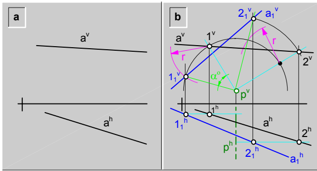
fig.245.\ Rotación de una recta.
