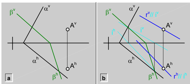
fig.162. Recta ( r ) paralela a dos planos ( \alpha y \beta )\ ejemplo.
