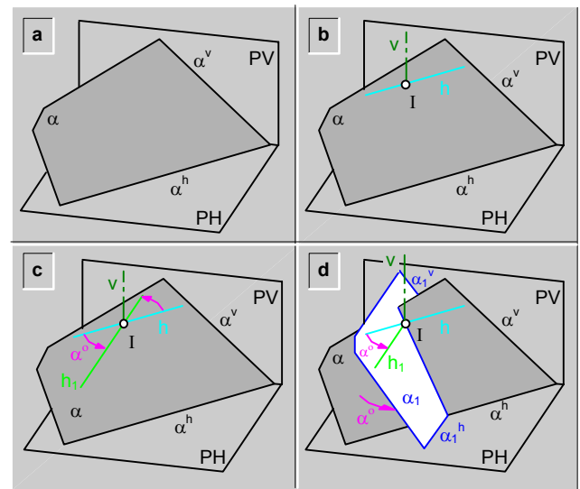
fig.254.\ Rotación de un plano a posición de punta.
