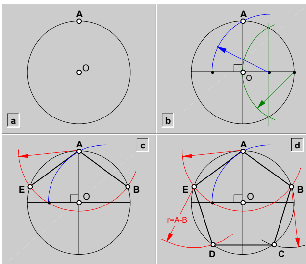
fig.29.\ Dibujo de un pentágono regular (ABCDE), conocido el vértice (A) y la circunferencia que lo circunscribe.
