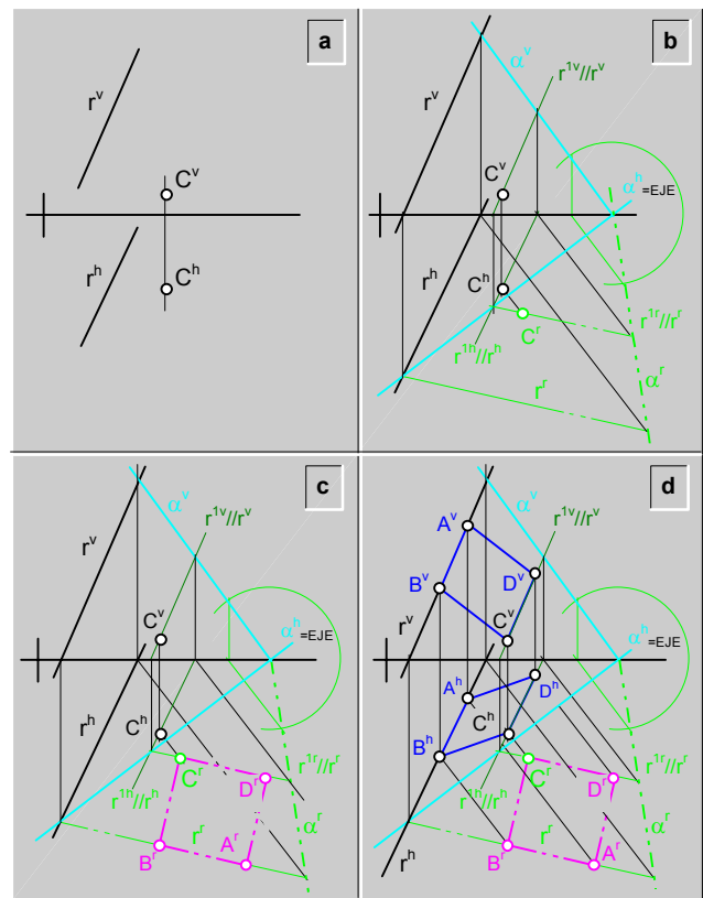
fig.238. \ Construcción de un cuadrado por rebatimiento previo de la traza vertical.
