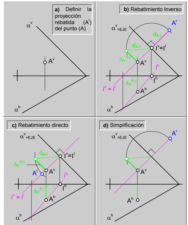
fig.224.\ Rebatimiento a través de la traza vertical.
