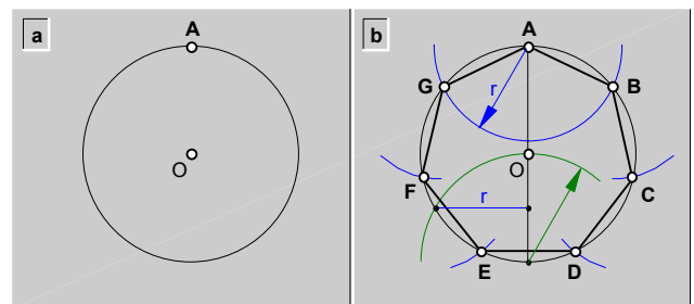
fig.33.\ Dibujo de un heptágono regular (ABCDEFG), conocido el vértice (A) y la circunferencia que lo circunscribe.
