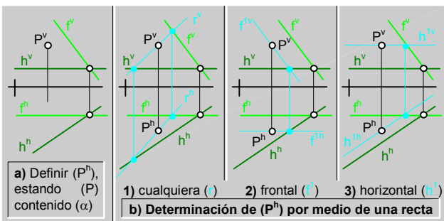
fig.133. \ Punto que pertenece a un plano definido por rectas características.
