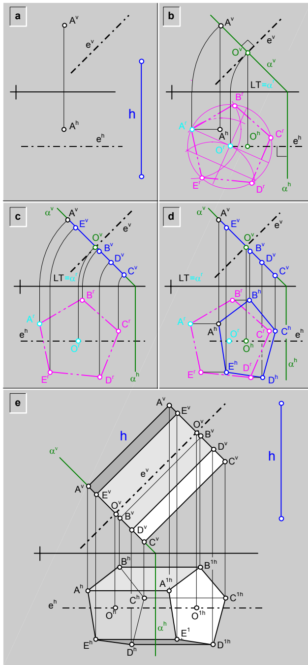
fig.304.1 Construcción de un prisma regular recto de base pentagonal (ABCDE), conocido: la altura (h); el vértice (A) de la base (ABCDE); y la recta (e) que contiene al eje ejemplo.
