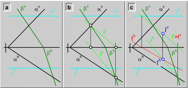
fig.156.\ Intersección (I) de tres planos\ ejemplo.
