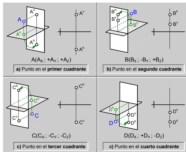
fig.69.\ Ubicación de un punto en un cuadrante.
