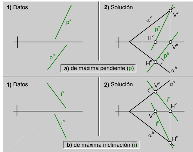
fig.177.\ Determinar las trazas del plano ( \alpha ) definido por la recta...
