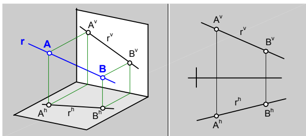
fig.83.\ Proyección diédrica de una recta.
