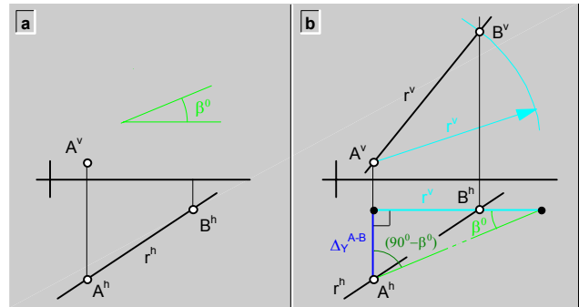
fig.107.\ Construcción de rectas (PH + β).
