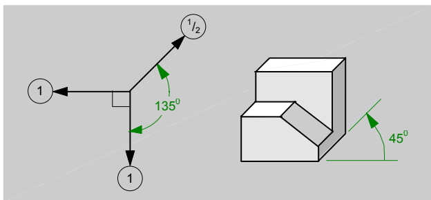
fig.56.\ Proyección de gabinete.
