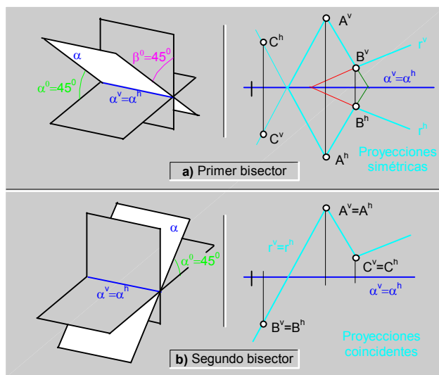
fig.139. Planos bisectores.
