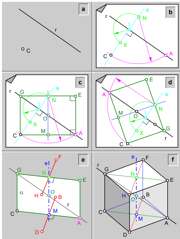
fig.291. Construcción de un cubo conocido un vértice y una recta que contiene a una diagonal mayor.
