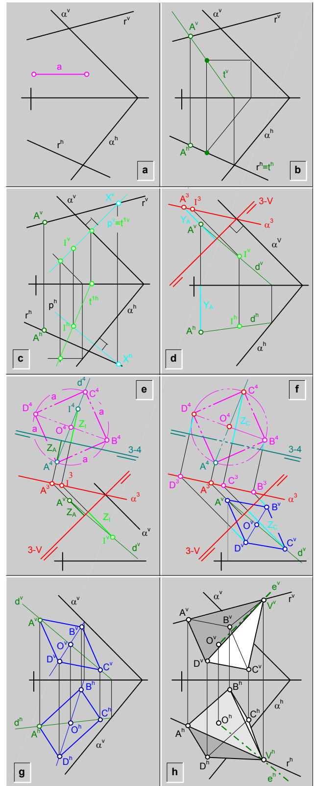
fig.297.1 Construcción de una pirámide regular recta, conocido el plano base; una recta que contiene a una arista principal; y la longitud de las aristas de la base\ ejemplo.
