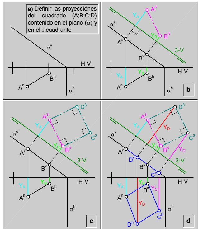
fig.266.1 Cambio del plano horizontal de proyección, para observar en posición horizontal a un plano de punta\ ejemplo.
