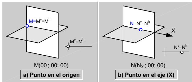
fig.72.\ Punto en el origen; punto en el eje (X) (línea de tierra).
