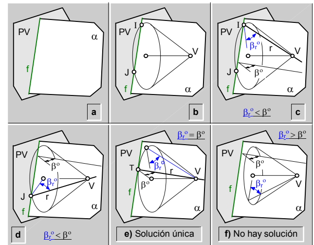
fig.213.\ Recta (r) contenida en un plano ( \alpha ) dado y que forma un ángulo ( \beta_r^\circ ) dado con el plano vertical de proyección.
