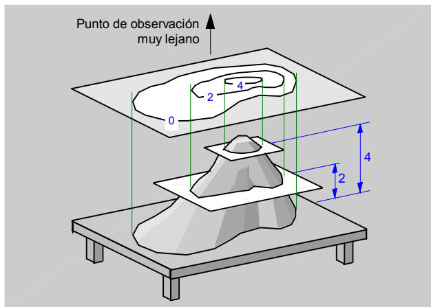
fig.48.\ Proyección acotada.
