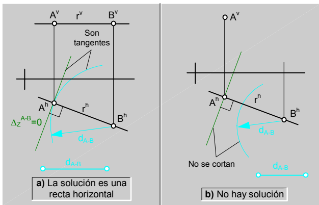
fig.110. Construcción de rectas (PH + VT) \ casos particulares.
