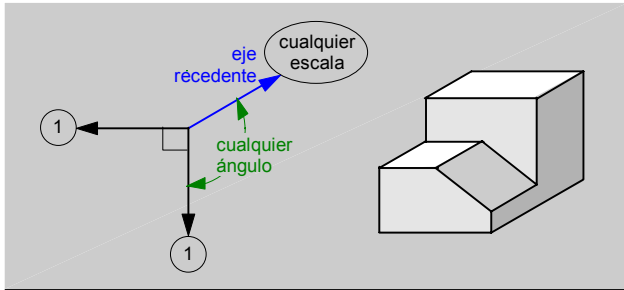
fig.54.\ Proyección oblicua.
