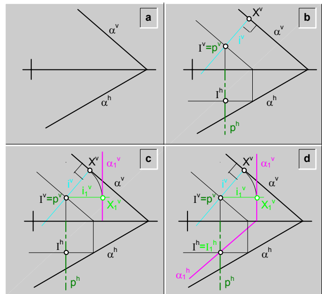
fig.248.\ Rotación de un plano a una posición vertical\ ejemplo.
