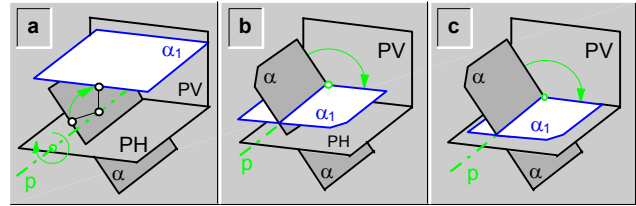
fig.258.\ Rotación de un plano ( \alpha ) en posición de punta a una posición ( \alpha_1 ) horizontal.
