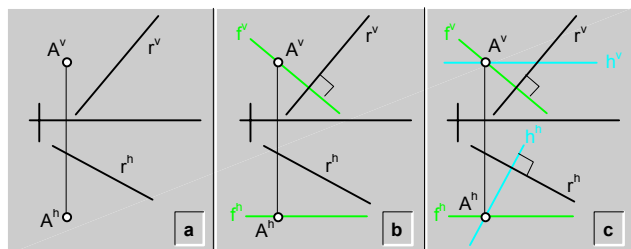
fig.172. Plano ( \alpha ), que contiene a un punto ( A ) y es perpendicular a una recta ( r ).
