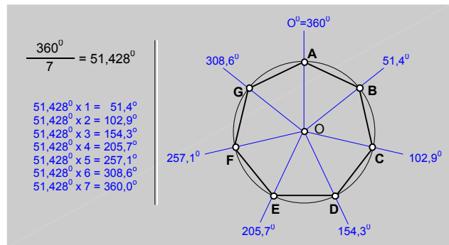
fig.36.1 Dibujo de un heptágono regular, (Método general).
