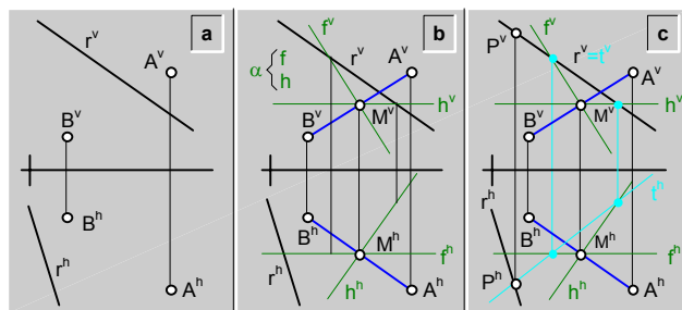
fig.200.\ Punto (P) que equidista de dos puntos (A y B) dados y se encuentra sobre una recta (r) dada \ ejemplo.
