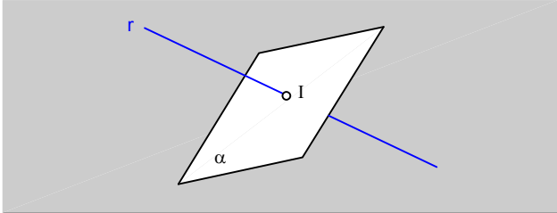
fig.140.\ Intersección ( I ) entre una recta ( r ) y un plano ( \alpha ).
