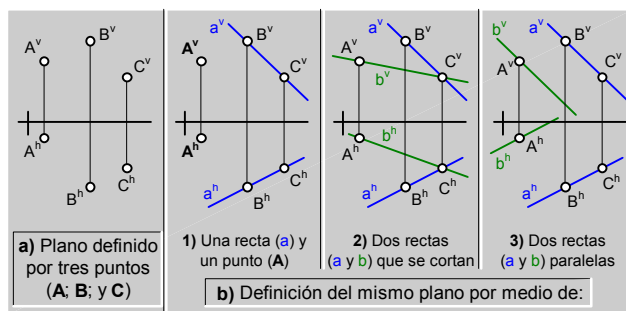
Fig.122.\ Cambio de la definición original de un plano.
