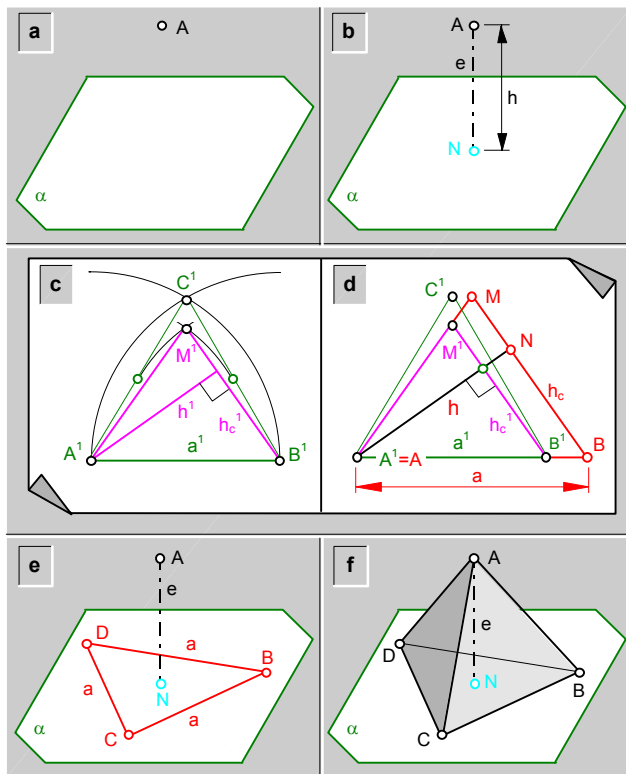
fig.283. \ Construcción de un tetraedro regular, conocido el plano que contiene a una cara y el vértice no contenido en este plano.
