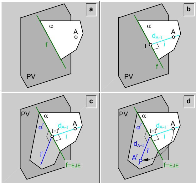
fig.223.\ Rebatimiento de un plano ( \alpha ) a través de su traza vertical (f).
