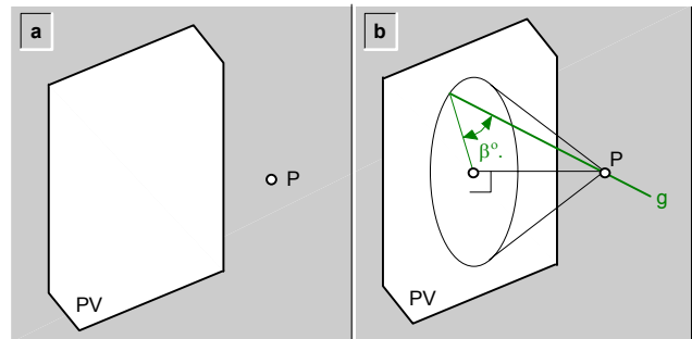
fig.205.\ Recta ( g ) que contiene a un punto ( P ) dado y forma un ángulo ( \beta^\circ ) dado con el plano vertical de proyección.
