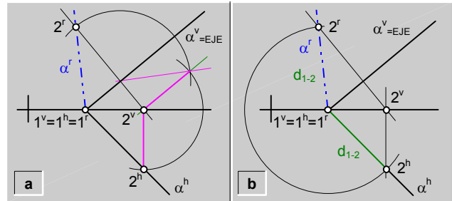
fig.226.1 Rebatimiento de la traza horizontal de un plano.
