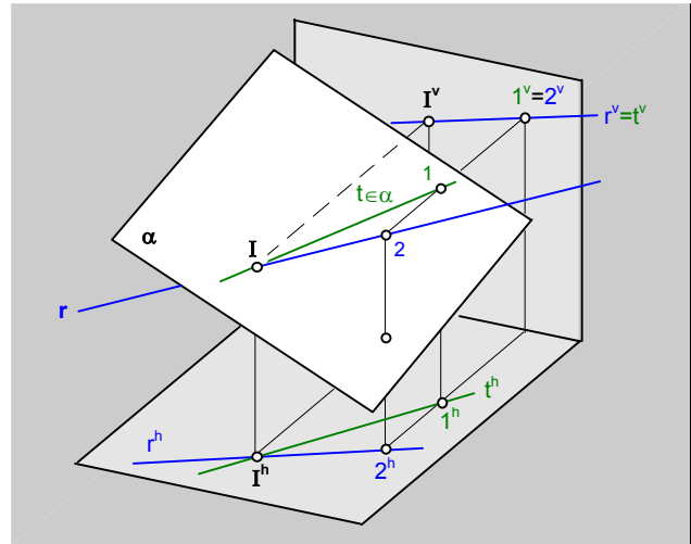
fig.142.\ Determinación de la intersección ( I ) entre una recta ( r ) y un plano ( \alpha ), tapando las proyecciones verticales ( r^v y t^v ) de las rectas ( r y t ).
