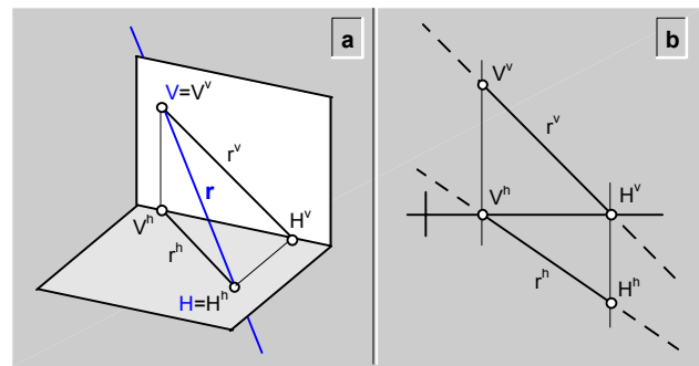
fig.86.\ Trazas de una recta.
