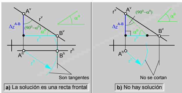
fig.106.\ Construcción de rectas (PV + α) \ casos particulares.
