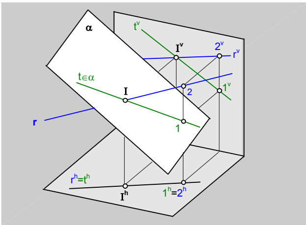
fig.141.\ Determinación de la intersección ( I ), entre recta ( r ) y plano ( \alpha ), tapando las proyecciones horizontales ( r^h y t^h ) de las rectas ( r y t ) .
