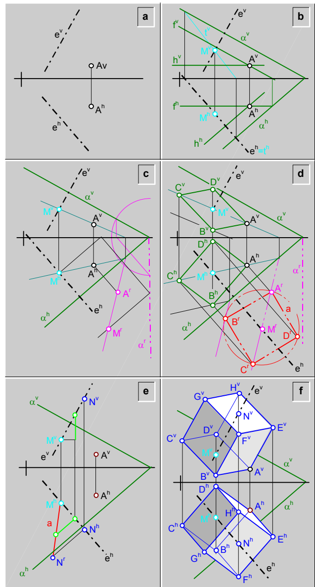
fig.290.\ Construcción de un cubo, conocido el vértice (A) y la recta (e) que contiene a un eje ejemplo.
