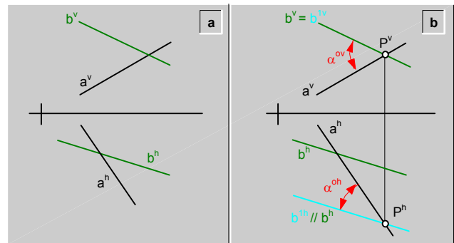
fig.192.\ Ángulo ( \alpha^\circ ) entre dos rectas (a y b) que se cruzan.
