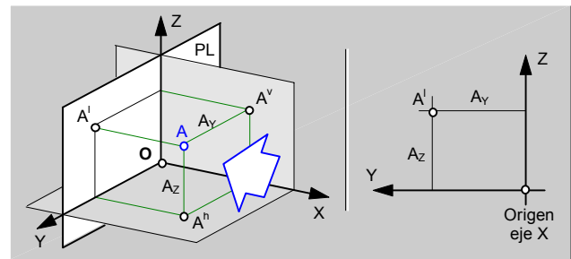
fig.75.\ Proyección lateral.
