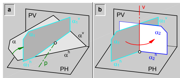
fig.252.\ Rotación de un plano a una posición frontal.
