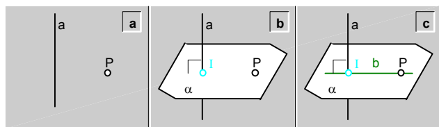
fig.173. Recta ( b ), que contiene a un punto ( P ), y es perpendicular a otra recta ( a ).
