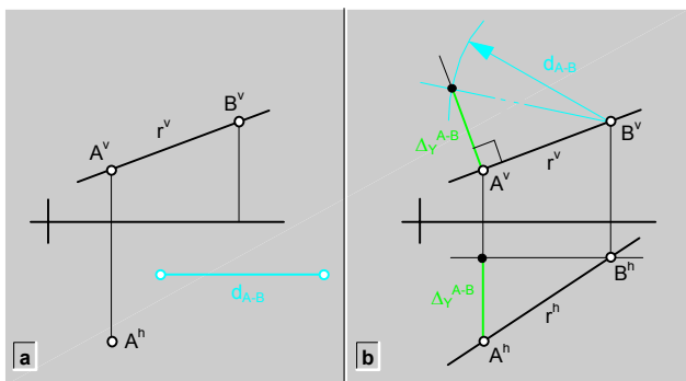
fig.111. Construcción de rectas (PV + VT).
