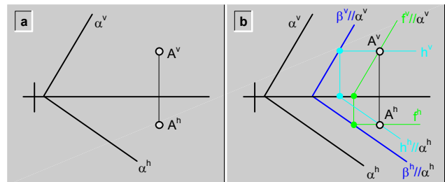
fig.165. Paralelismo entre planos\ ejemplo 2.
