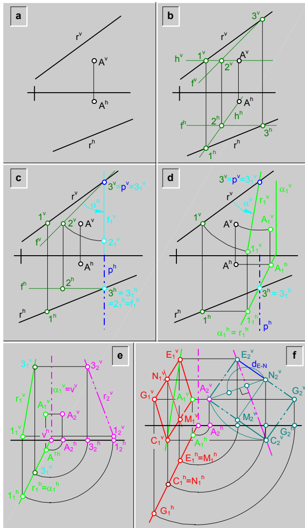
fig.292.\ Construcción de un cubo conocido un vértice (A) y una recta (r) que contiene a una diagonal mayor (E-C)\ ejemplo.
