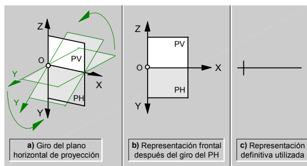
fig.67. Dibujo en proyección diédrica.
