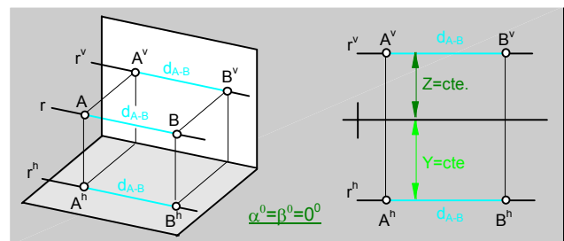
fig.98.\ Recta paralela a la línea de tierra.
