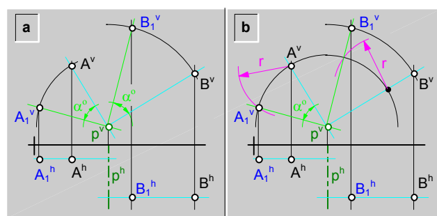
fig.244.\ Rotación simultánea de varios puntos.
