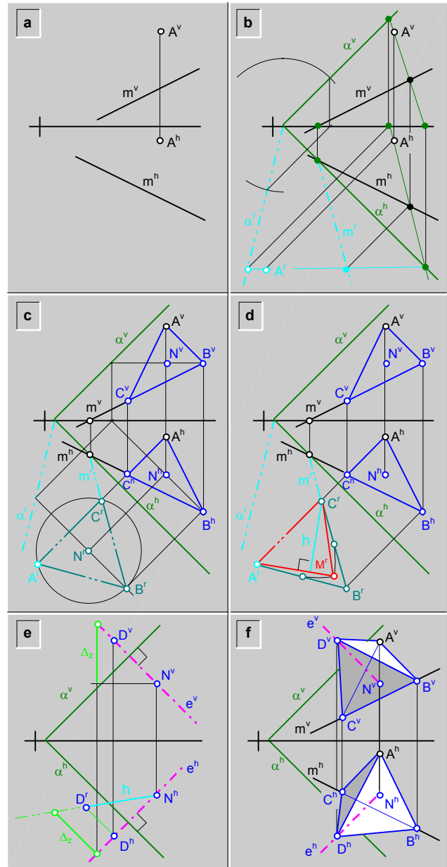
fig.282.\ Construcción de un tetraedro regular conocido un vértice y una recta que contiene a una arista ejemplo.
