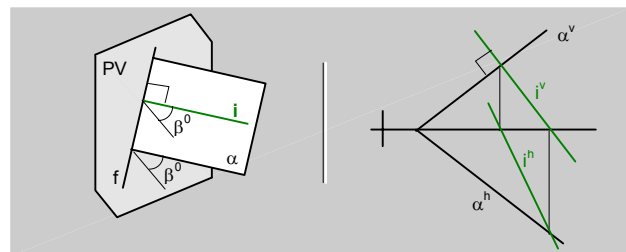
fig.176. Recta ( i ) de máxima inclinación de un plano ( \alpha ).
