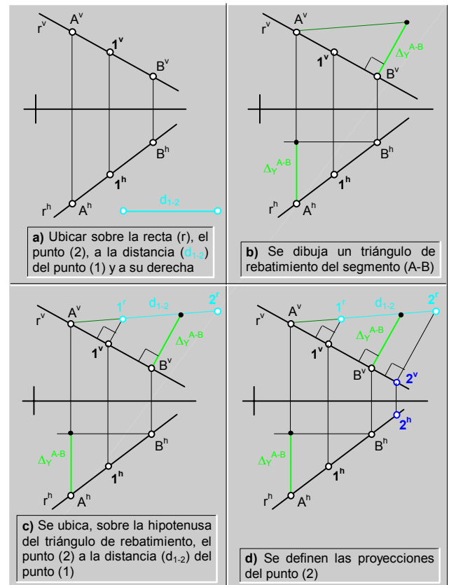
fig.93. \ Medición de distancias en rectas.
