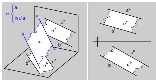
Fig.120.\ Plano ( \alpha ) definido por dos rectas (a y b) paralelas.
