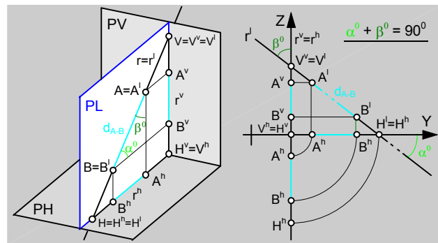
fig.102.\ Recta de perfil.
