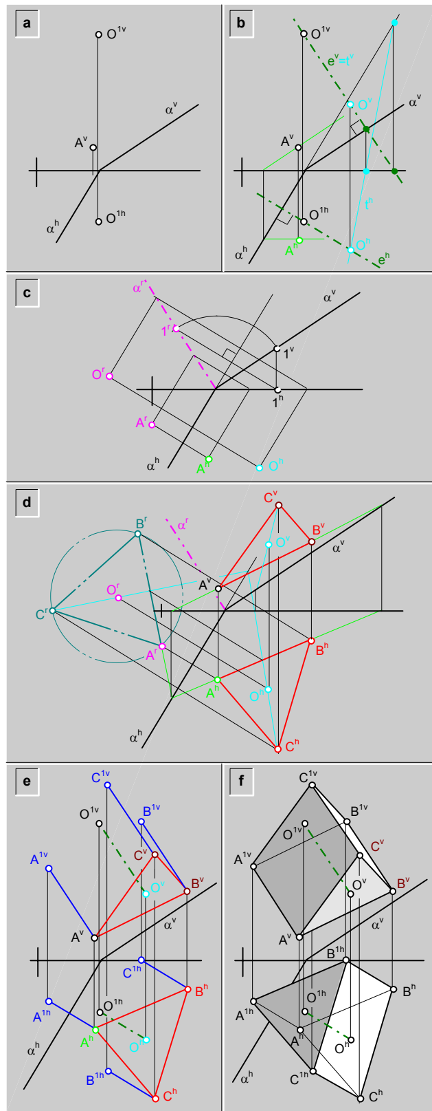
fig.302.\ Construcción de un prisma regular recto, de base triangular (ABC) contenida en el plano ( \alpha ), siendo ( O^1 ) el centro de la otra base ( A^1B^1C^1 ) ejemplo.
