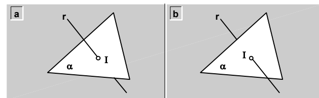
fig.147.\ Intersección entre una recta y un plano VISIBILIDAD.
