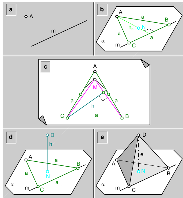
fig.281.\ Construcción de un tetraedro regular con vértice (A) y arista (B-C) en la recta (m).
