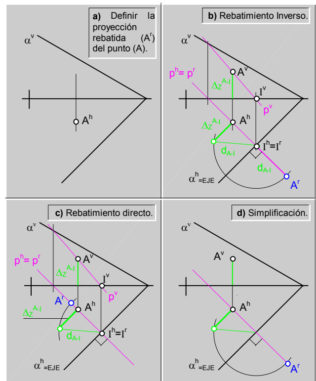
fig.219. \ Rebatimiento a través de la traza horizontal.
