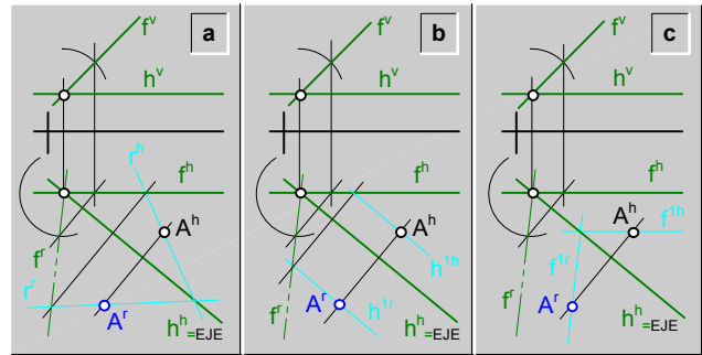
fig.232.1 Rebatimiento de un punto (A) de un plano ( \alpha ) por medio del rebatimiento previo de una recta frontal (f).
