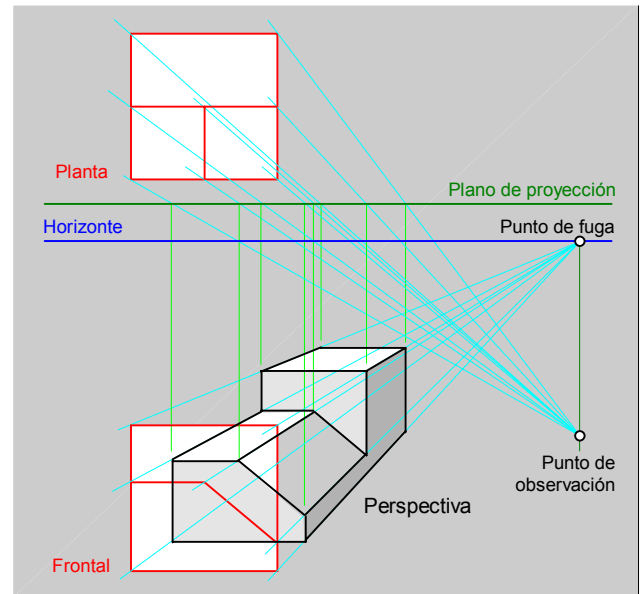
fig.62.\ Dibujo de una perspectiva de un punto de fuga.
