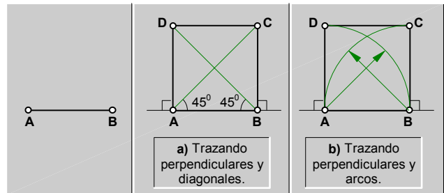
fig.26.\ Dibujo de un cuadrado (ABCD), conocido el lado (AB).
