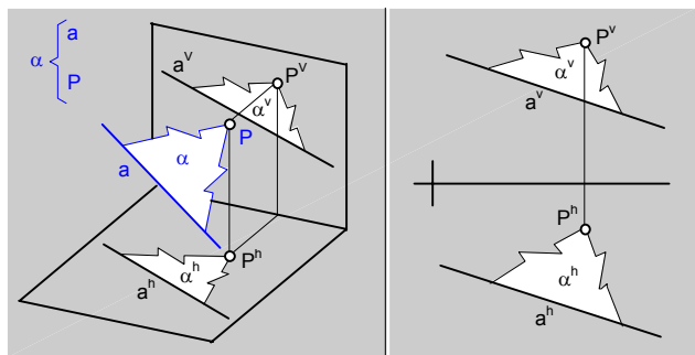
Fig.118.\ Plano ( \alpha ) definido por una recta (a) y un punto (P).
