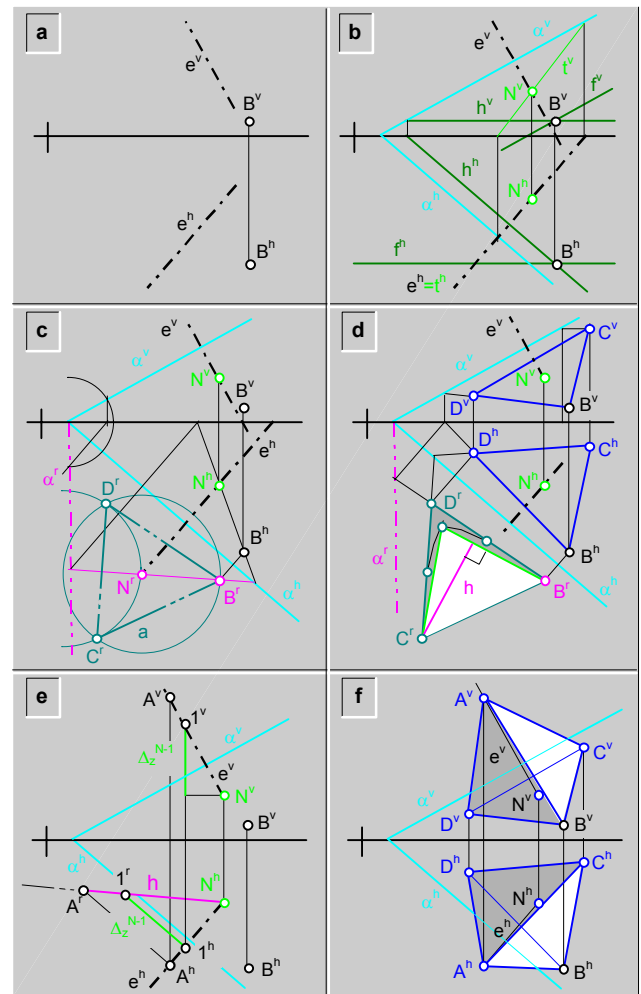
fig.280.\ Construcción de un tetraedro regular, conocido un vértice y una recta que contiene al eje.
