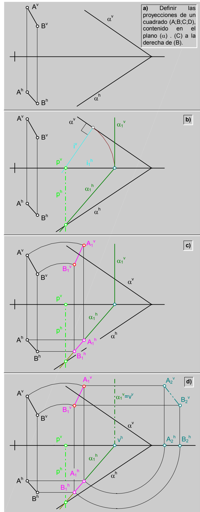
fig.253. Rotación de un plano a una posición frontal \ ejemplo.
