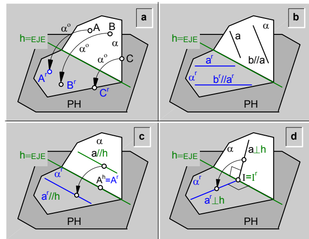
fig.216.\ Generalidades del rebatimiento.
