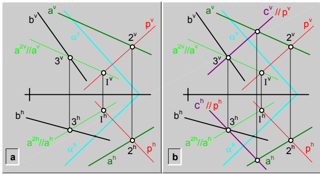
fig.190.\ Perpendicular común (c) a dos rectas (a y b) que se cruzan\ ejemplo.
