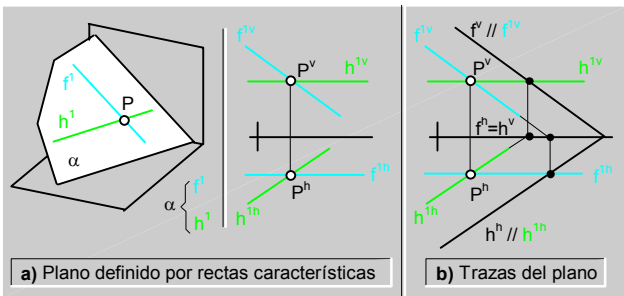
fig.132. \ Plano ( \alpha ) definido por rectas ( f^1 y h^1 ) características.
