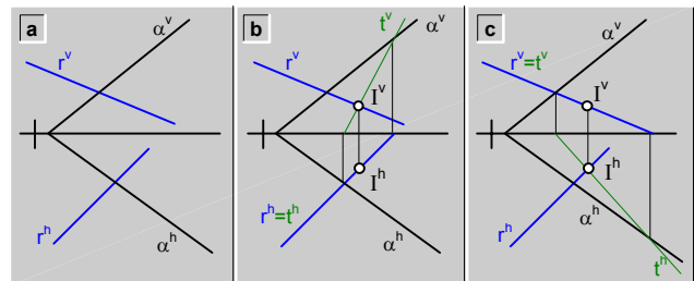
fig.143.\ Intersección ( I ) de la recta ( r ) con el plano ( \alpha ) definido por trazas.
