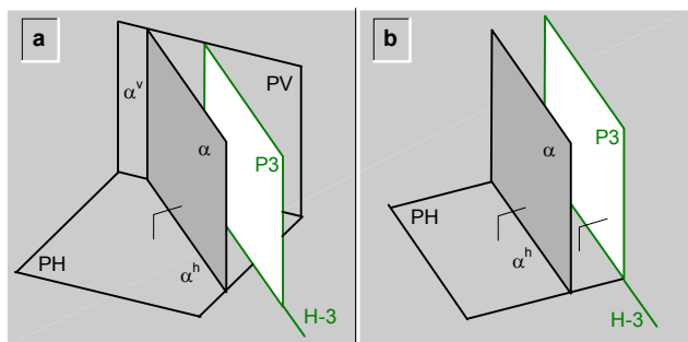
fig.271.\ Cambio del plano vertical de proyección para observar en posición frontal a un plano vertical.
