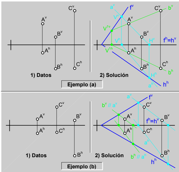
fig.128. Determinación de las trazas de un plano ejemplos.
