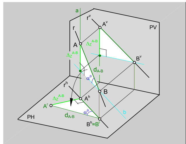
fig.89. \ Triángulo de rebatimiento horizontal.
