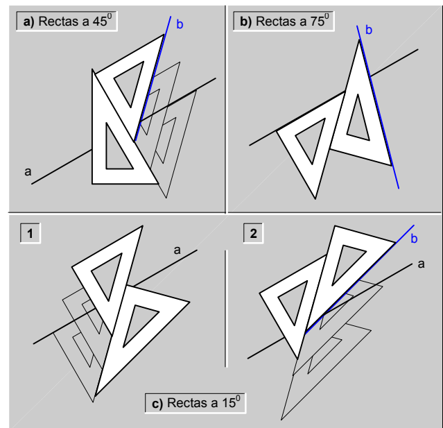
fig.19.\ Trazado de rectas a 45^\circ ; 75^\circ y 15^\circ .
