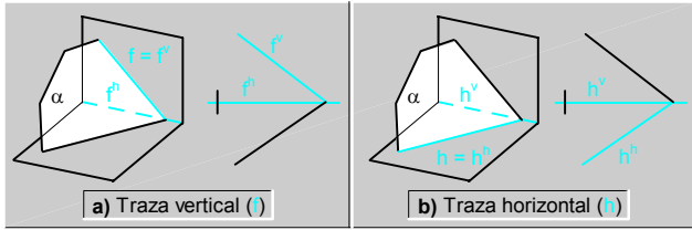
Fig.126. Trazas de un plano.
