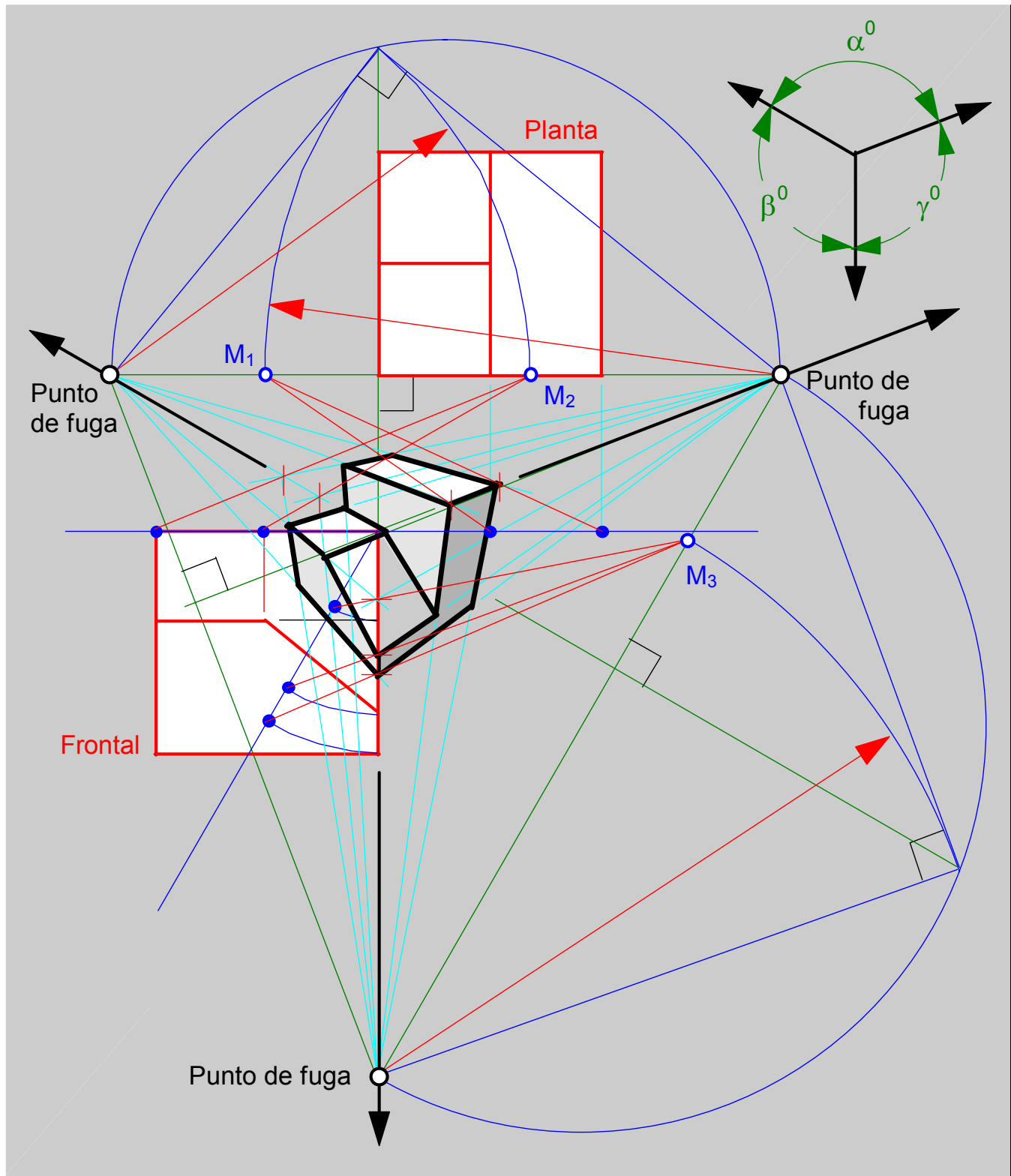
fig.64.\ Dibujo de una perspectiva de tres puntos de fuga.
