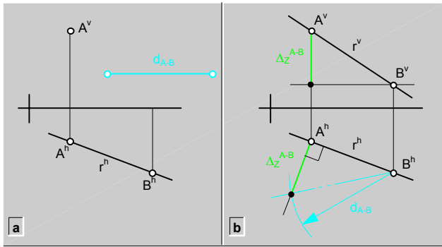
fig.109. Construcción de rectas (PH + VT).
