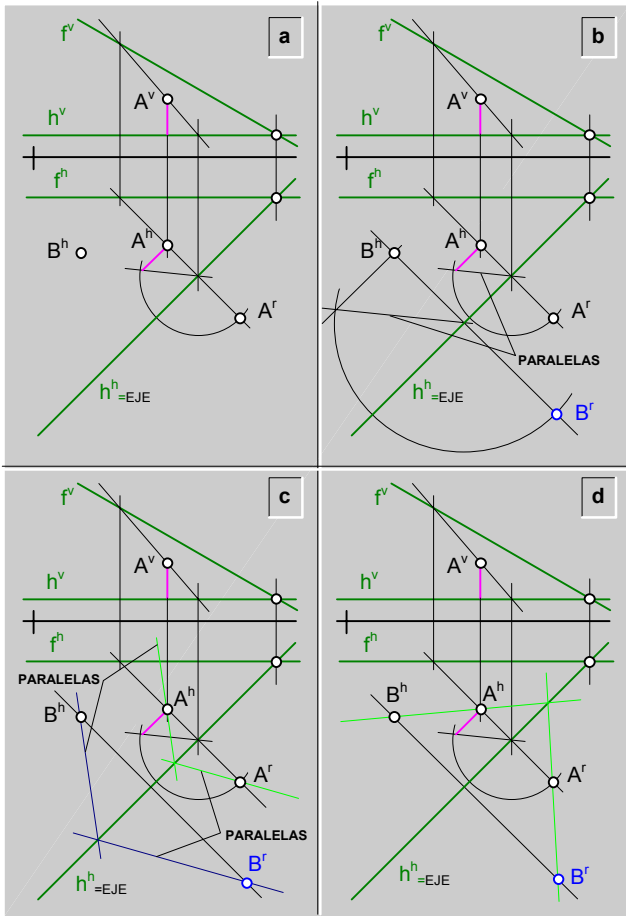
fig.230.1 Rebatimiento de varios puntos.
