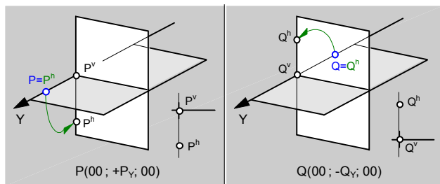
fig.73.\ Punto en el eje (Y).
