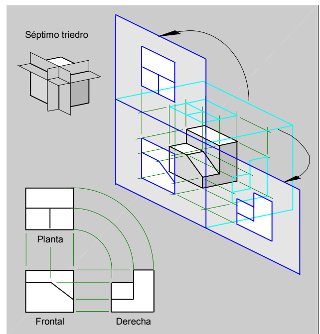
fig.46.\ Proyección en vistas múltiples en el séptimo triedro.
