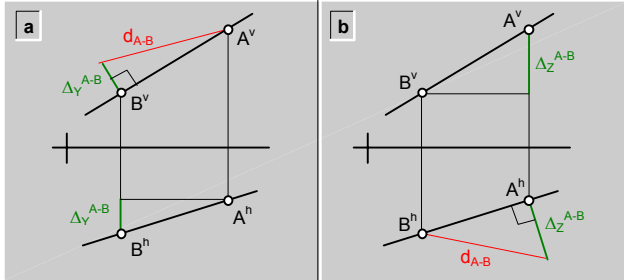
fig.182.\ Distancia ( d_{A-B} ) entre dos puntos (A y B).
