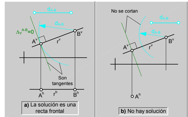
fig.112. Construcción de rectas (PV + VT) \ casos particulares.
