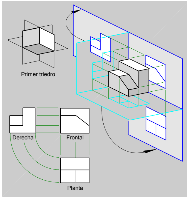
fig.47.\ Proyección en vistas múltiples en el primer triedro.
