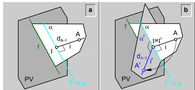
fig.233.1 Rebatimiento a través de una recta característica frontal ( f^1 ) de un plano ( \alpha ).
