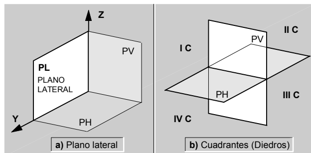
fig.66. Plano lateral / Cuadrantes.
