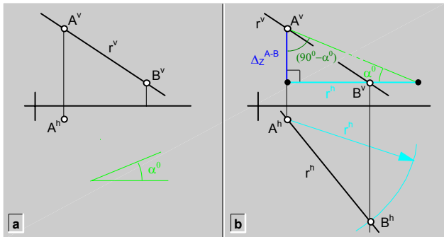
fig.105.\ Construcción de rectas (PV + α).
