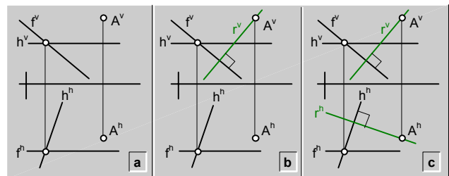
fig.171. \ Recta (r), que contiene a un punto (A) y es perpendicular a un plano ( \alpha ), definido por rectas características
