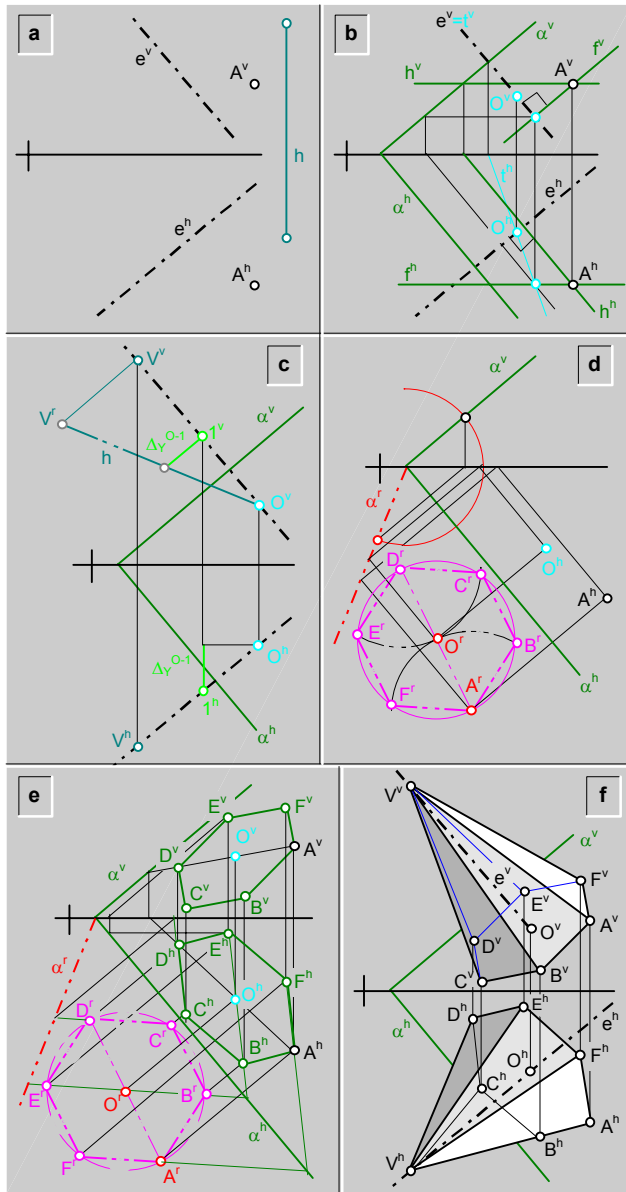
fig.295.1 Construcción de una pirámide regular recta conocido: la altura (h); un vértice (A) de la base; y una recta (e) que contiene al eje\ ejemplo.
