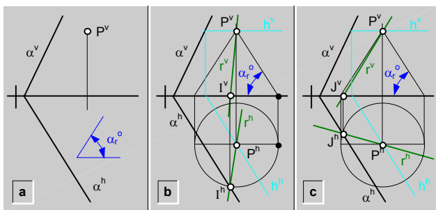
fig.212.\ Recta (r) contenida en un plano ( \alpha ) dado y que forma un ángulo ( \alpha_r^\circ ) dado con el plano horizontal de proyección\ ejemplo.
