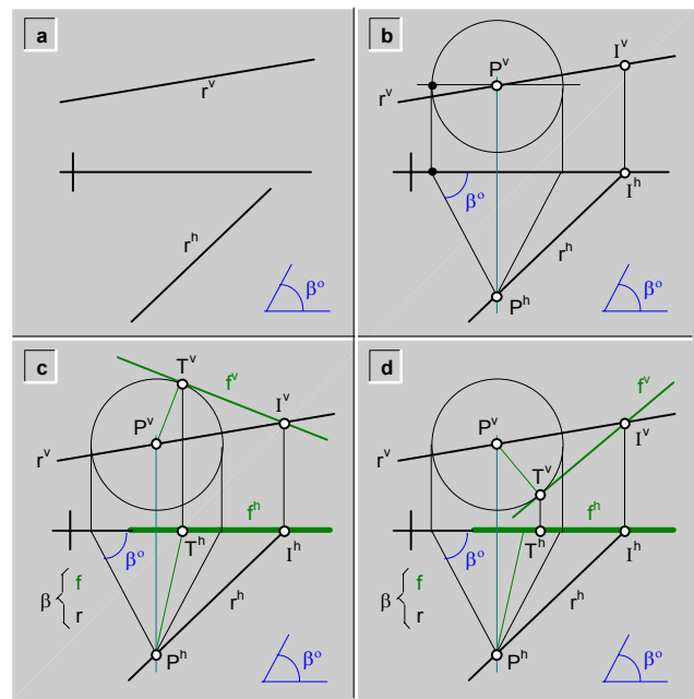
fig.210.\ Plano ( \alpha ) que contiene a una recta ( r ) dada y forma un ángulo ( \beta^\circ ) dado con el plano vertical de proyección\ ejemplo.
