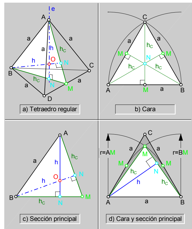
fig.278.\ Tetraedro regular.
