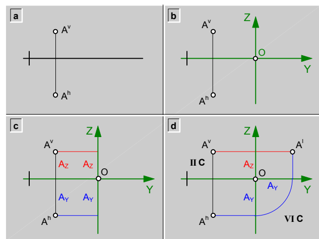
fig.78.1 Determinación de la proyección lateral de un punto (A), a partir de su doble proyección ortogonal.
