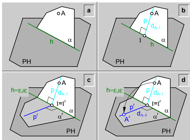
fig.218. \ Rebatimiento de un plano ( \alpha ) a través de su traza horizontal (h).
