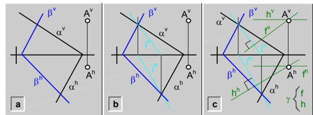
fig.181.\ Plano ( \gamma ), que contiene a un punto ( A ), y es perpendicular a los planos ( \alpha y \beta ).
