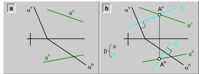
fig.179.\ Plano ( \beta ), que contiene a una recta ( a ), y es paralelo a otro plano ( \alpha ).
