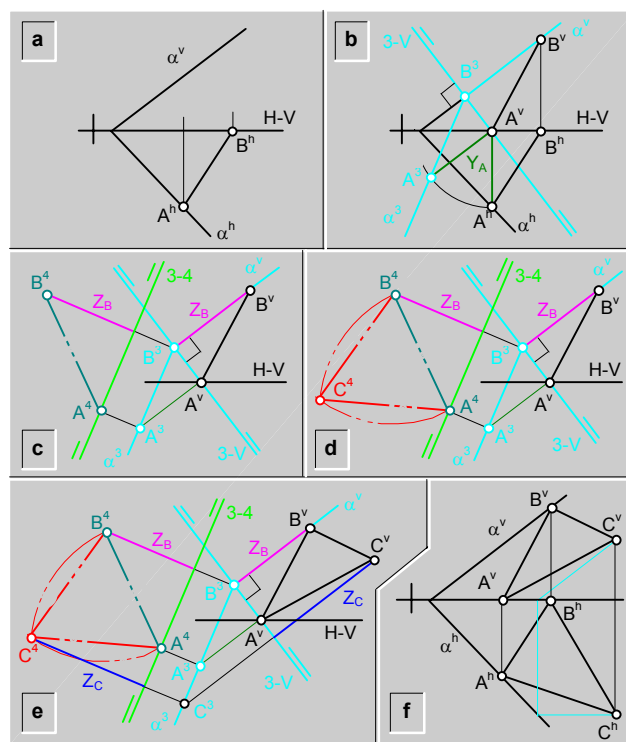
fig.274.\ Observación de un plano en posición frontal, por medio de dos cambios de plano de proyección\ ejemplo.
