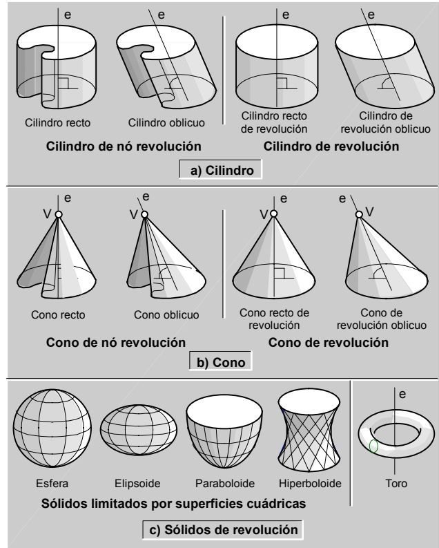
fig.14.1 Cuerpos redondos.
