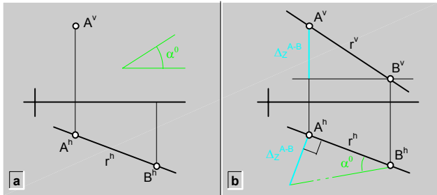
fig.104.\ Construcción de rectas (PH + α).
