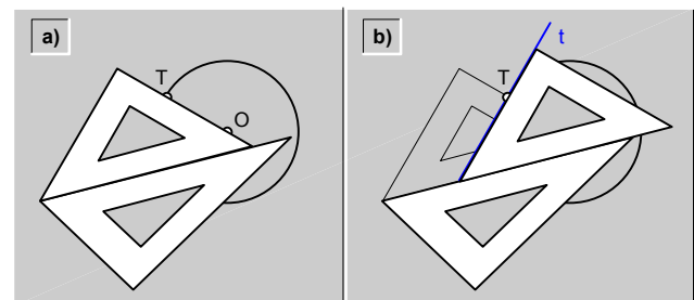
fig.20.\ Recta (t), tangente a una circunferencia, en un punto (T) de ella.
