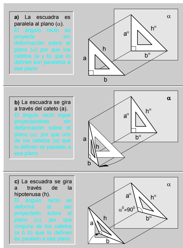
fig.166. Propiedad proyectiva del ángulo recto.
