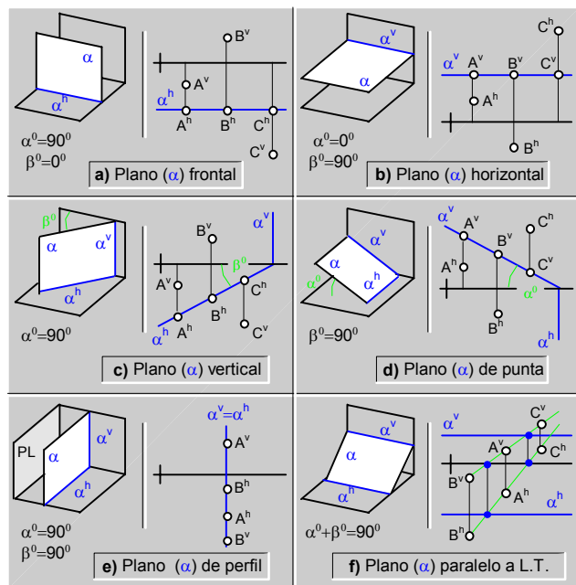
fig.137. Planos en posiciones particulares.
