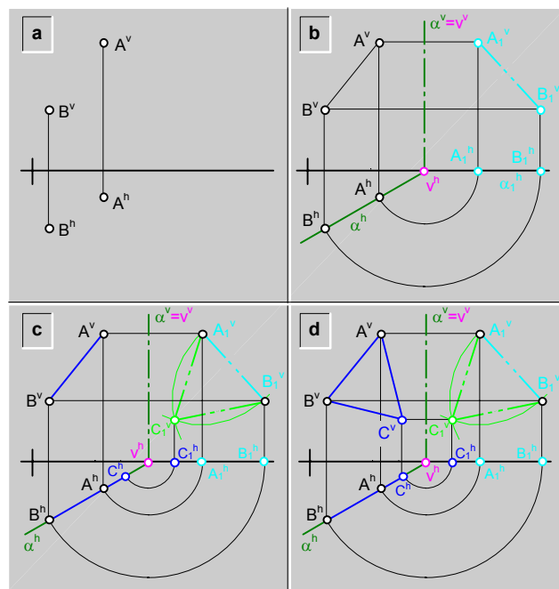
fig.251.\ Rotación de un plano vertical a una posición frontal.
