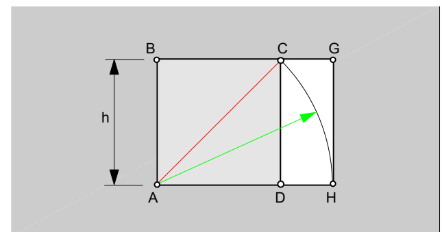
fig.287.\ Dibujo de la sección principal (ABGH), a partir de la cara (ABCD).
