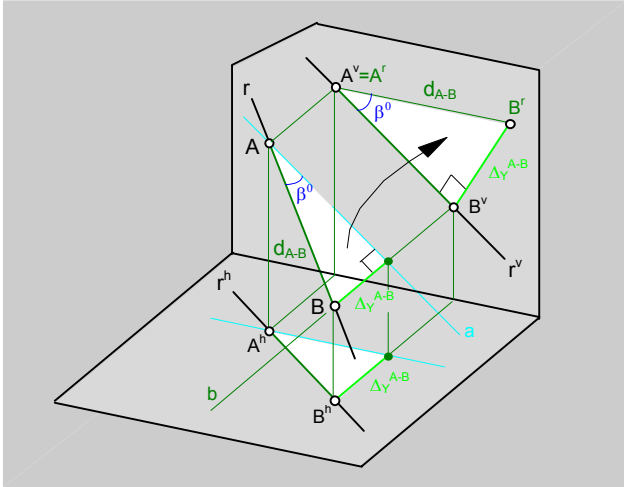
fig.90. \ Triángulo de rebatimiento vertical.
