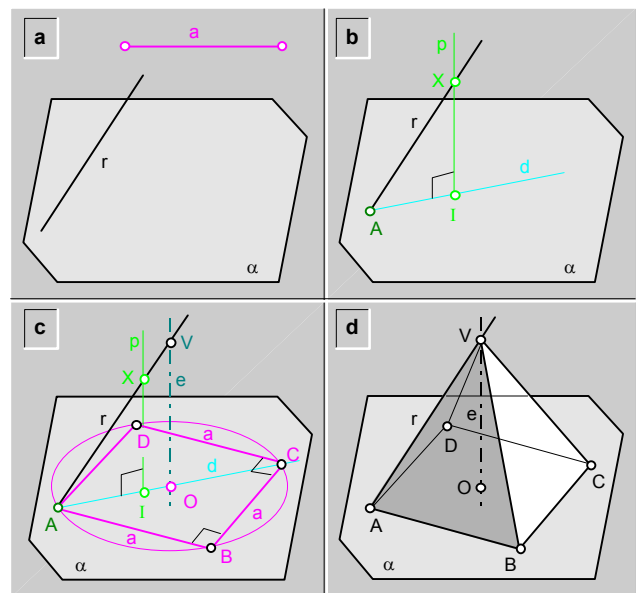
fig.296.1 Construcción de una pirámide regular recta, conocido el plano de la base; una recta que contiene a una arista principal; y la longitud (a) de las aristas de la base.
