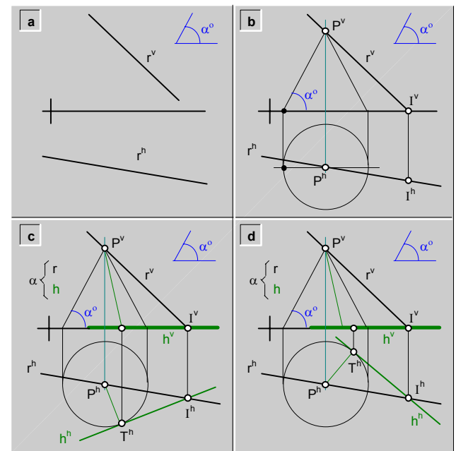
fig.208.\ Plano ( \alpha ) que contiene a una recta (r) dada y forma un ángulo ( \alpha^\circ ) dado con el plano horizontal de proyección\ ejemplo.
