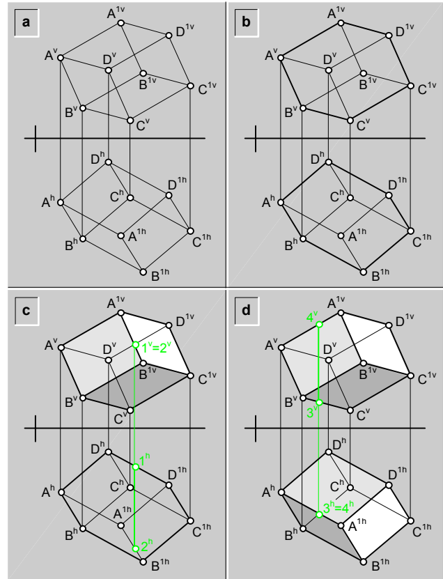
fig.276.\ Definición de la visibilidad de un poliedro.
