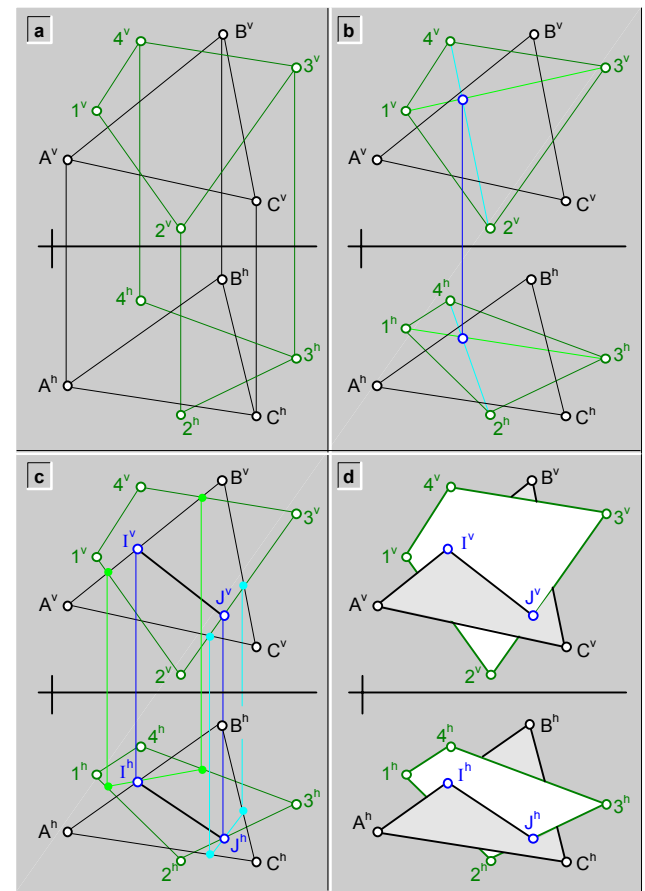
fig.154.\ Intersección y visibilidad de dos planos\ ejemplo.
