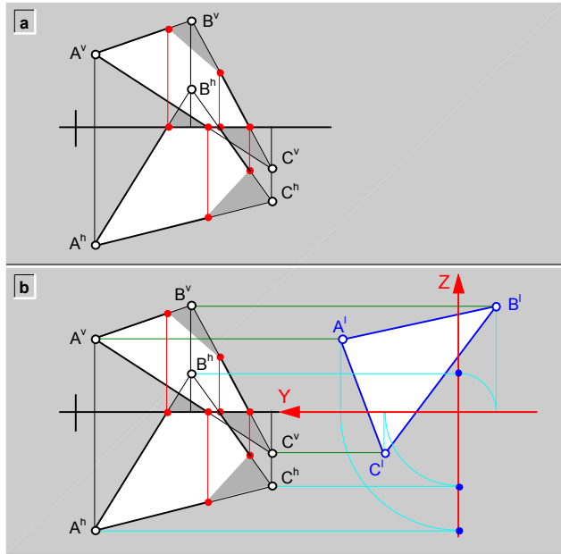
fig.80.1 Proyección lateral de un triángulo (A;B;C).
