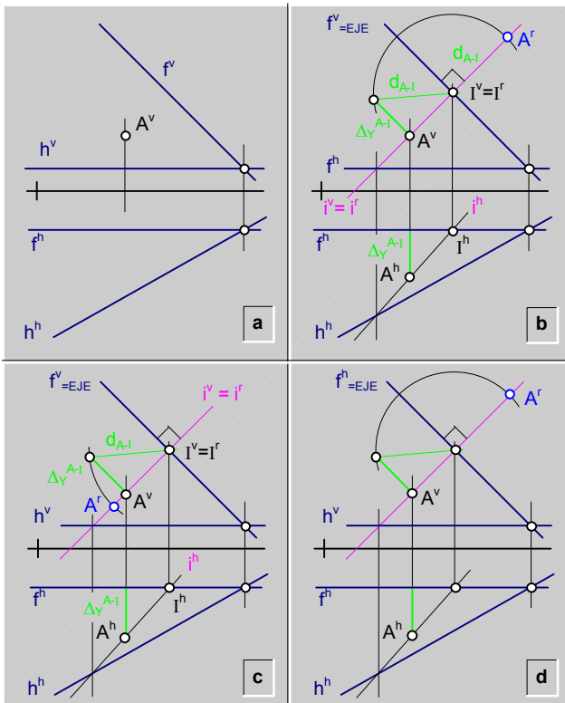
fig.234.\ Rebatimiento alrededor de una recta característica frontal ( f ) de un plano ( \alpha ) ejemplo.
