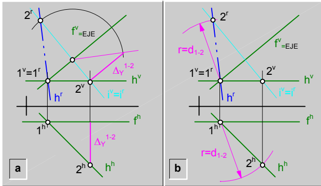
fig.236. \ Rebatiendo de una horizontal ( h ) de un plano ( \alpha ).
