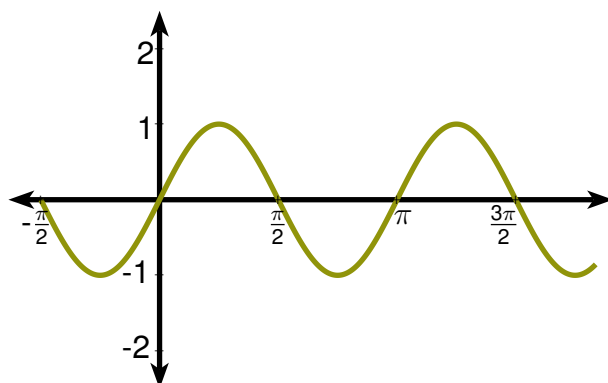
(III) Gráfico de \sin(2x) .
