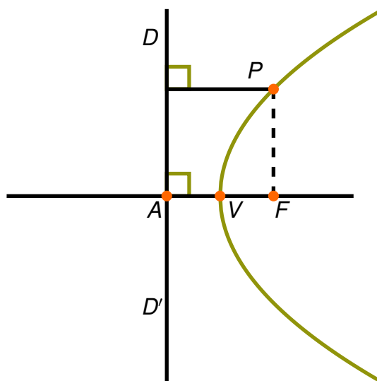
Figura 9.4: Elementos de una parábola
