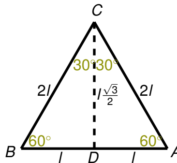
Figura 4.2: Triángulo equilátero.
