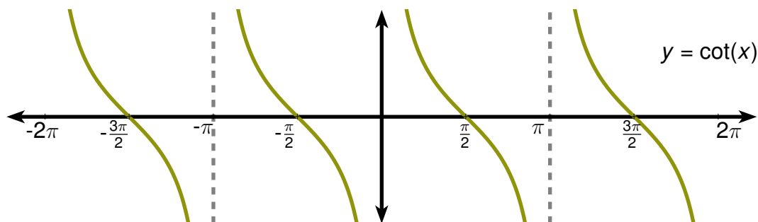
Figura 4.10: Gráfico de la función cotangente.
