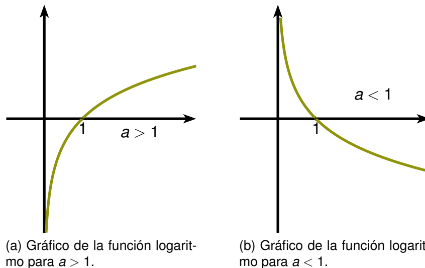
Figura 8.3: Gráfico de la función logaritmo.
