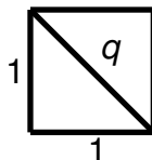
Figura 2.11: Cuadrado de lado unitario.
