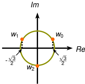
Figura 7.3: Gráfico de las raíces cúbicas de z = i .
