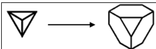
Fig. 30: Del tetraedro se obtiene el tetraedro truncado
