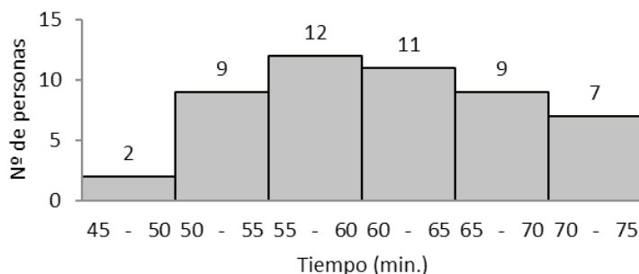
Gráfica 1. Distribución del número de personas según el tiempo que tardan en realizar una actividad. (Elaboración propia).
