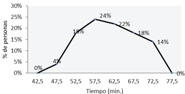
Gráfica 4. Comportamiento del número de personas según el tiempo que tardan en realizar una actividad. (Elaboración propia).
