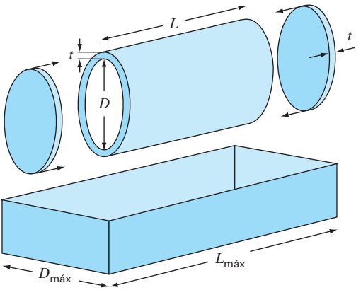
FIGURA 16.1 Parámetros para determinar las dimensiones óptimas de un tanque cilíndrico.
