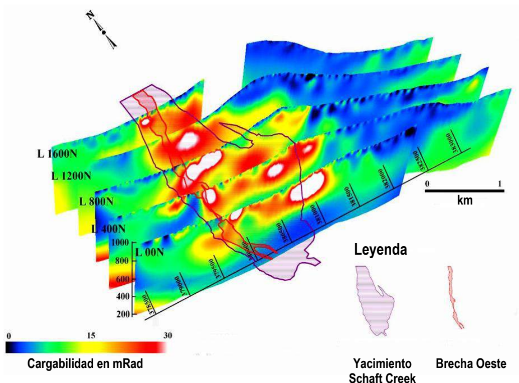
Secciones IP a lo largo del yacimiento de Cu-Au-Mo-Ag Shaft Creek (Columbia Británica, Canadá) (Copper Fox Metals Inc., 2010). Note el excelente perfilado del yacimiento mediante polarización inducida.
