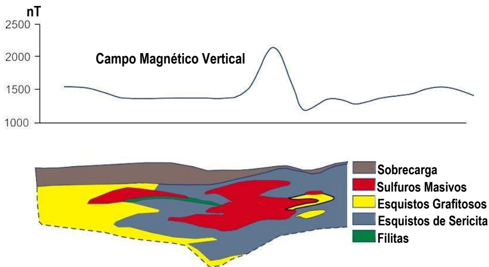
Anomalía magnética en el yacimiento de sulfuros masivos de Vangorda (Yukón, Canadá) (Ford et al., 2008).
