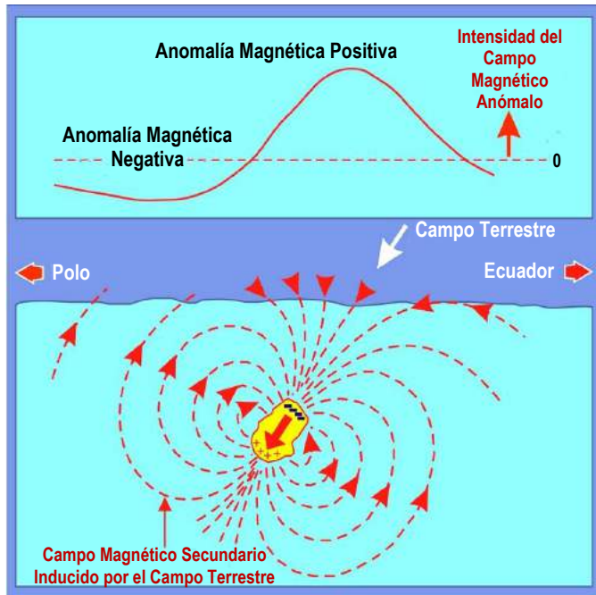
La magnetización inducida en un cuerpo geológico produce localmente una anomalía magnética positiva y una anomalía magnética negativa subsidiaria (Ford et al., 2008).
