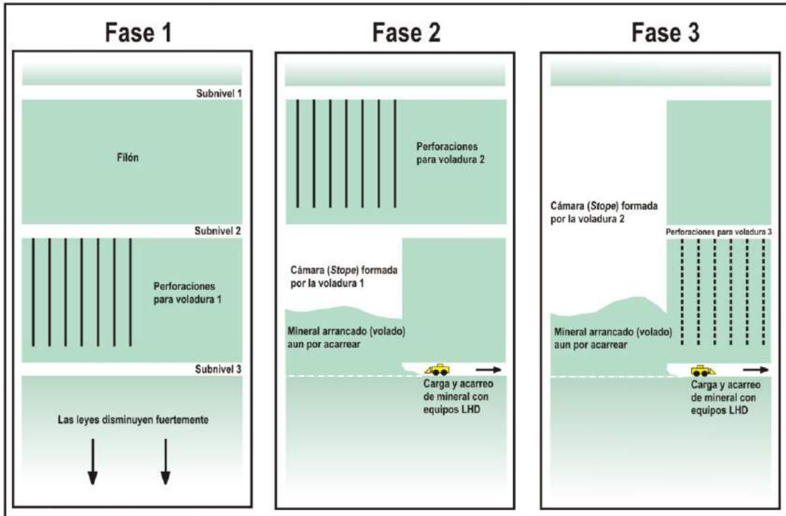
Esquema simplificado (explicado por fases) del método de Hundimiento por Subniveles. En este caso consideramos un filón y perforaciones verticales. La sección pasa "a lo largo" del filón.
