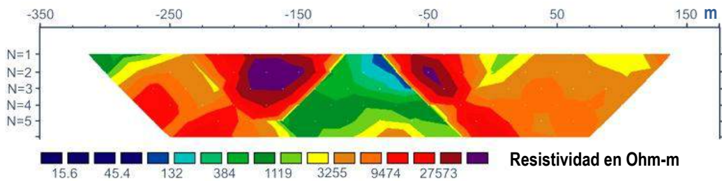
Ejemplo de perfil de resistividad (Ford et al., 2008).
