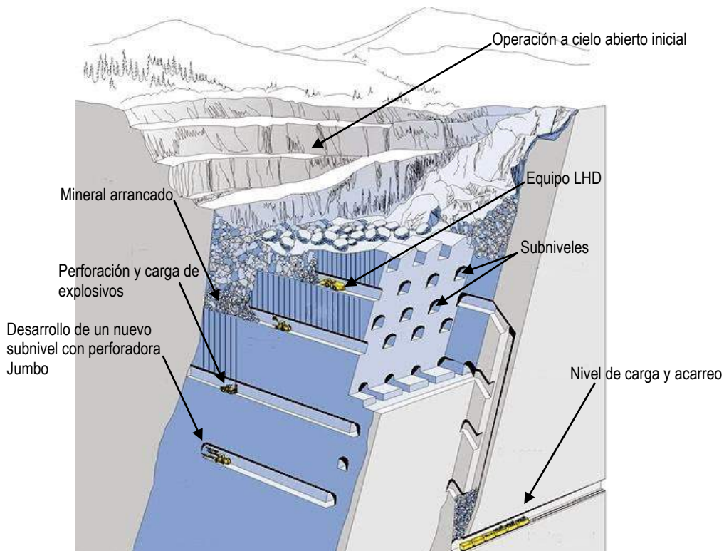
Diagrama simplificado que muestra una operación minera por el método de Pisos de Hundimiento ( Sublevel Caving ) (imagen 12 ) (Atlas Copco, 2007).
