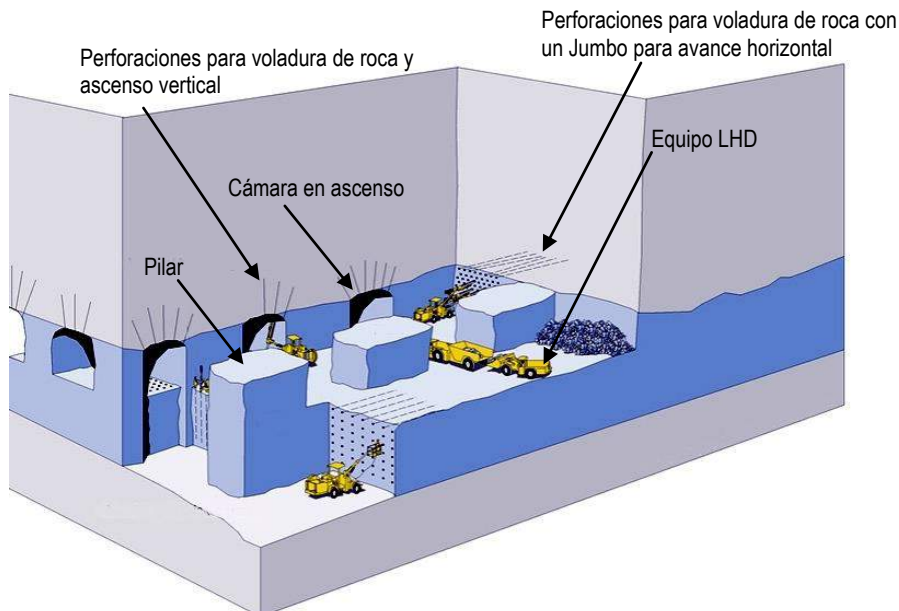
Diagrama simplificado que muestra una operación minera por el método de Cámaras y Pilares ( Room and Pillar ) (imagen 9 ) (Atlas Copco, 2007).
