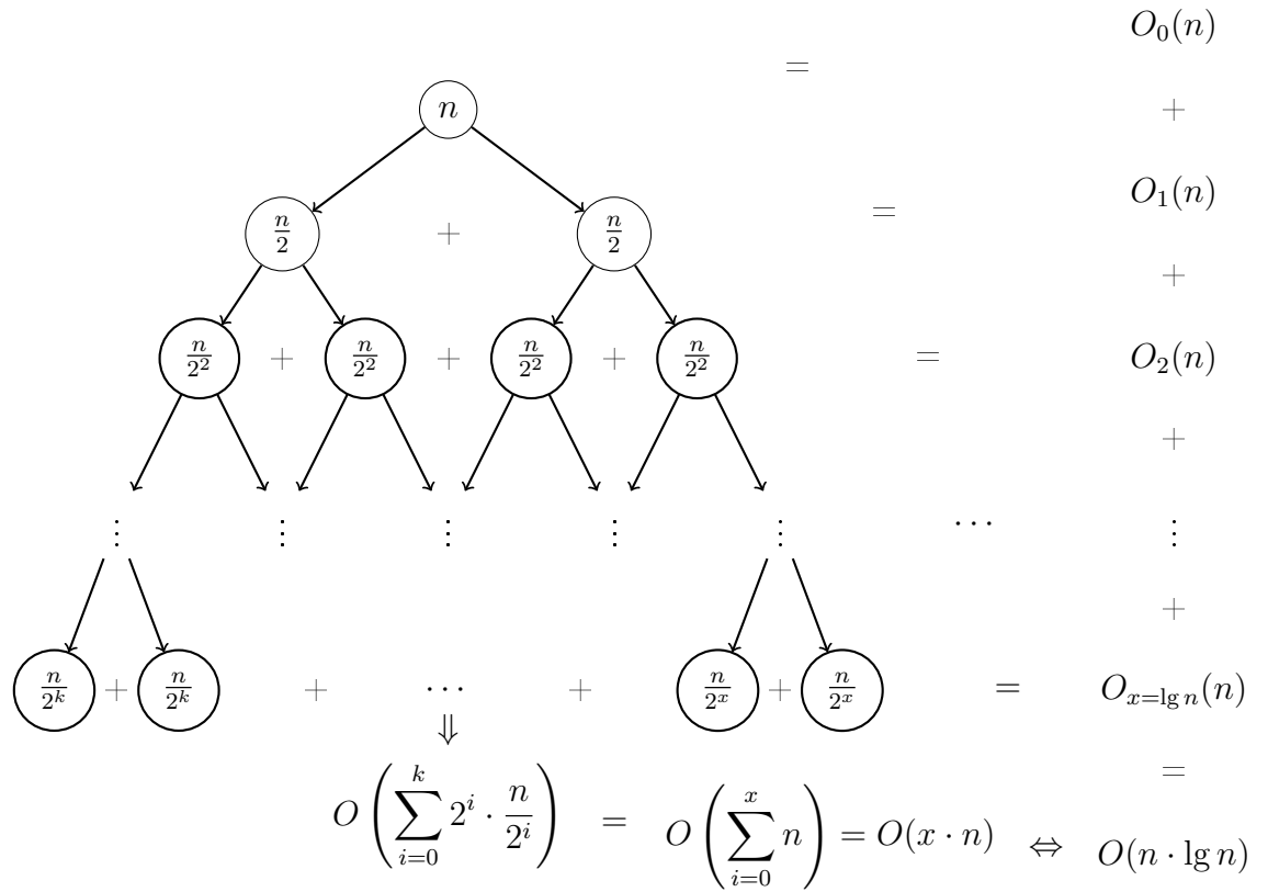
Figura 12.1: Rendimiento del ordenamiento por mezcla
