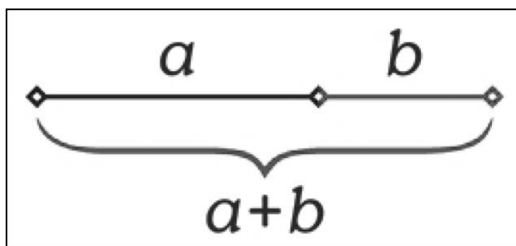
(14.2). La proporción áurea en una línea.
