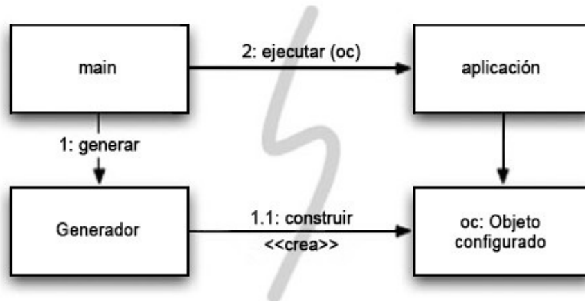
Figura 11.1. Separación de la construcción en main() .
