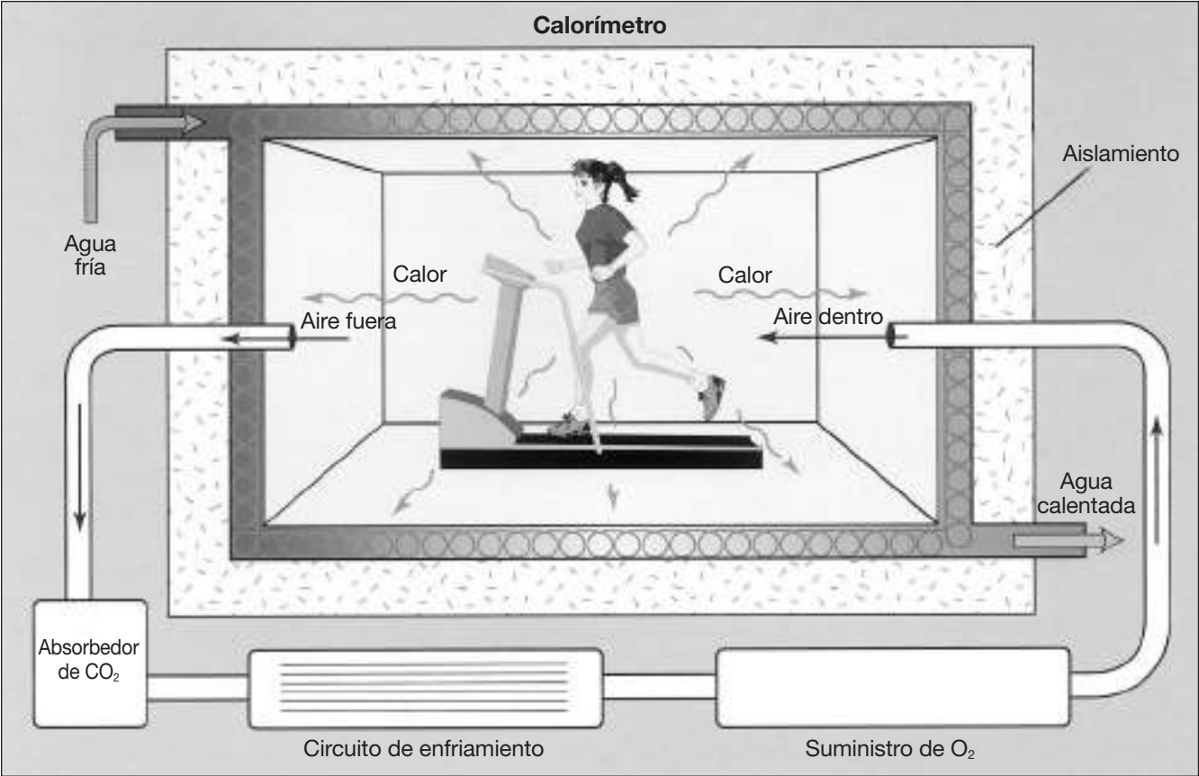
Figura 5.10 Una cámara calorimétrica.
