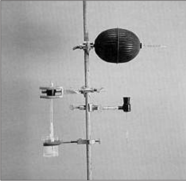
Figura 11.8 Aparato con un globo y una bombilla húmeda para medir la temperatura.
