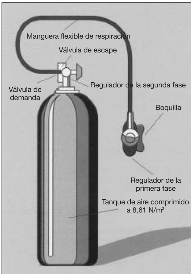
Figura 12.7. Sistema de escafandra autónoma de circuito abierto a la demanda.
