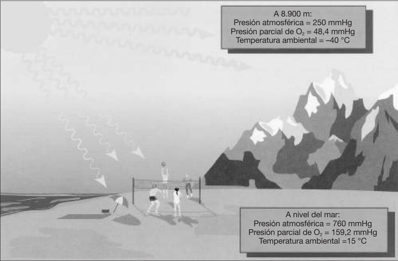
Figura 12.1 Diferencias en las condiciones atmosféricas a nivel del mar y a una altitud de 8.900 m.
