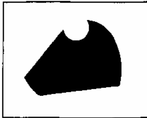
FIGURA IV. 1. Representación muy esquemática de un conjunto recursivo.
