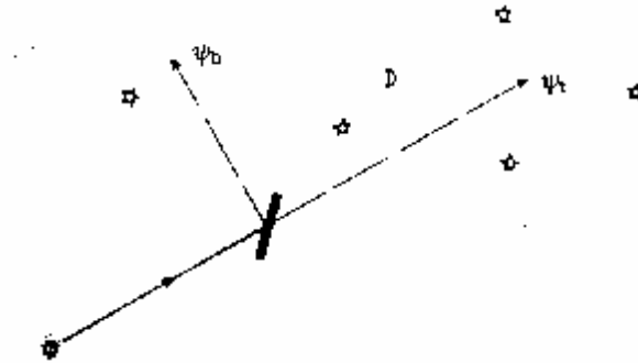
FIGURA VI. 17. Los dos picos de una función de onda podrían estar a años luz de distancia. Esto puede conseguirse por medio de un espejo semirreflectante.
