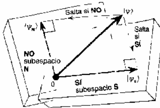
FIGURA VI.23. Reducción del vector de estado. Una medición sí/no puede describirse en términos de un par de subespacios S y N que son complementos ortogonales entre sí. En la medición el estado |y\rangle salta a su proyección sobre uno u otro de estos subespacios, con probabilidades dadas por el factor en que decrece el cuadrado de la longitud del vector de estado en la proyección.
