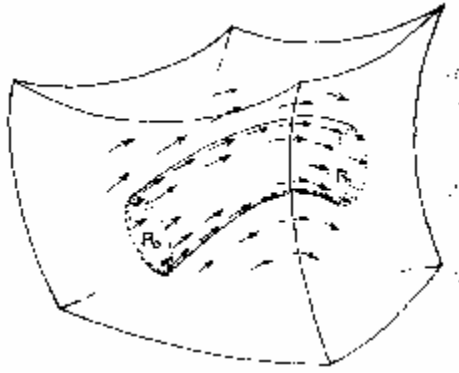
FIGURA V.13. A medida que pasa el tiempo, una región de estados de fase R_0 es arrastrada a lo largo del campo de vectores hacia una nueva región R_t . Esto representará la evolución temporal de una alternativa particular para nuestro dispositivo.
