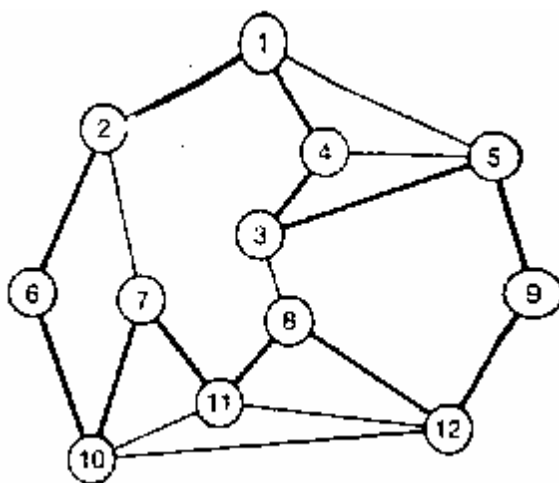
FIGURA IV. 14. Un grafo con un círculo hamiltoniano indicado: líneas más oscuras. Existe un círculo hamiltoniano más que el lector puede tratar de localizar.
