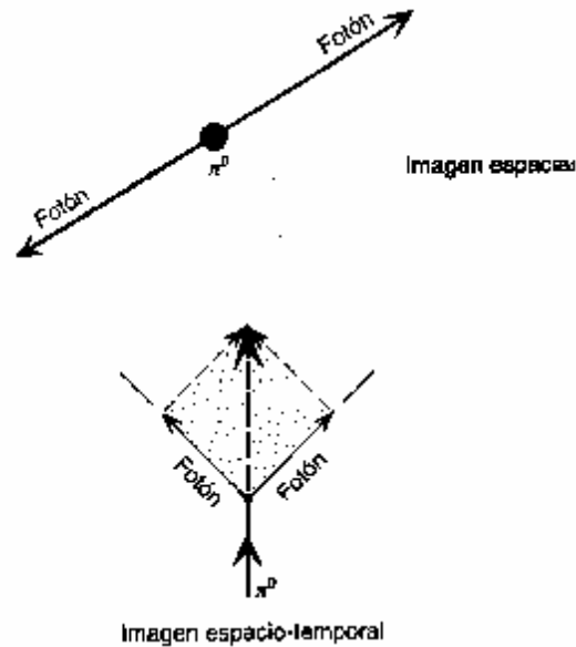
FIGURA V.36. Un mesón p^0 con masa se desintegra en dos fotones sin masa. La imagen espacio-temporal muestra cómo el cuadrivector energía-momento se conserva: el cuadrivector del mesón p^0 es la suma de los cuadrivectores de los dos fotones sumados según la ley del paralelogramo (representado sombreado).
