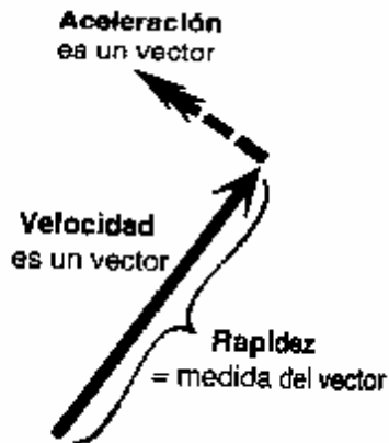
FIGURA V.4. Velocidad, celeridad y aceleración.
