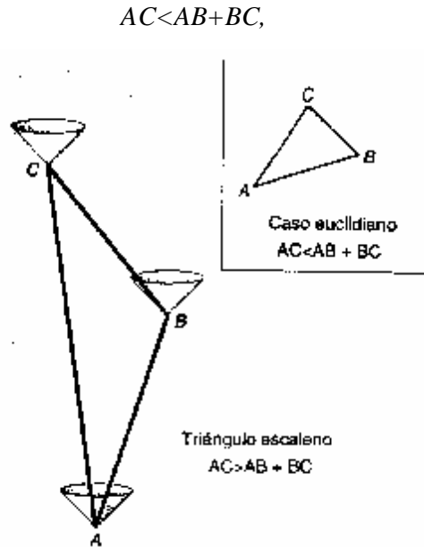
FIGURA V.19. La llamada "paradoja de los gemelos" de la relatividad especial se comprende en términos de una desigualdad triangular minkowskiana. (Se da también el caso euclidiano para fines de comparación.)
