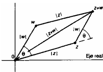
FIGURA VI.9. Geometría relativa al término correctivo 2|w||z|\cos q del módulo al cuadrado de la suma de dos amplitudes.
