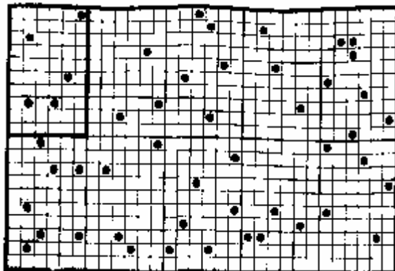
FIGURA VII.4. Modelo para un gas en una caja: cierto número de minúsculas bolas se distribuye entre un número mucho mayor de celdas. Una décima parte de las celdas está etiquetada como especiales. Estas son las recuadradas en la esquina superior izquierda.
