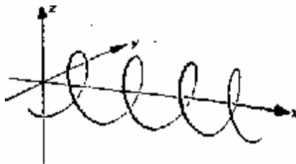
FIGURA VI.11. Un estado de momento tiene una curva y que es un sacacorchos.
