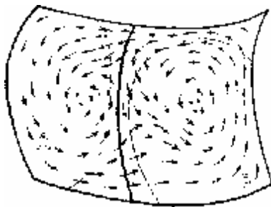
FIGURA VIII.5. El "flujo hamiltoniano" del contenido de la caja de Hawking (compárese con fig. V. 11). Las líneas de flujo que cruzan de A a B representan el colapso en un agujero negro, y las que cruzan de B a A representan la desaparición de un agujero negro por evaporación.
