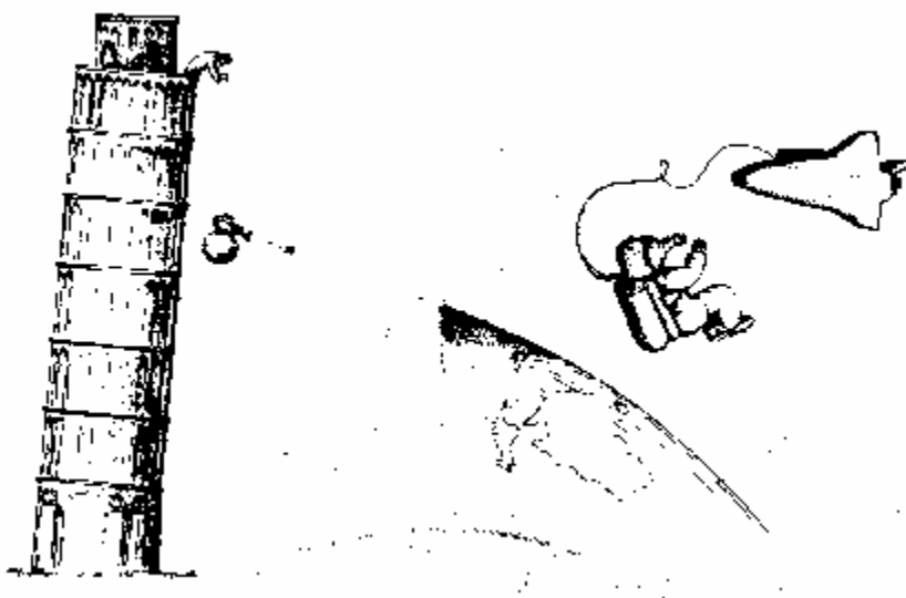
FIGURA V.23. Galileo dejando caer dos Piedras (y una videocámara) desde la torre inclinada de Pisa.
