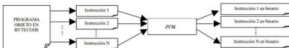
Fig. 5. La máquina virtual de Java (JVM) interpreta el bytecode durante la ejecución del programa.
