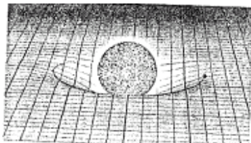
Figura 3.5 La Tierra se mantiene en órbita alrededor del Sol porque rueda por un valle situado en la estructura del espacio. Dicho de una manera más precisa, recorre una ‘trayectoria de resistencia mínima’ en la región distorsionada que rodea al Sol.
