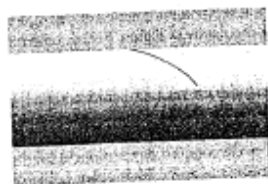
Figura 8.5 Un ser lineal puede ver directamente en el interior del cuerpo de otro cuando Linealandia se expande dentro del universo de la manguera.
