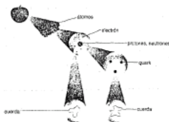
Figura 1.1 La materia está compuesta por átomos, que a su vez están hechos de quarks y electrones. Según la teoría de cuerdas, todas estas partículas son en realidad diminutos bucles de cuerdas vibrantes.
