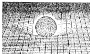
Figura 3.4 Un cuerpo provisto de masa, como el Sol, hace que la estructura del espacio se alabee, en cierto modo igual que el efecto de una bola de jugar a los bolos colocada sobre una membrana de goma.
