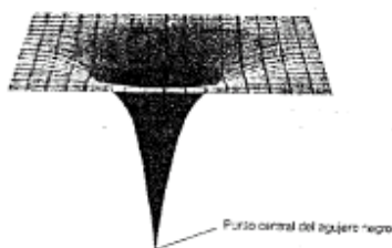
Figura 3.7 Un agujero negro hace que la estructura del espacio-tiempo que lo rodea se alabee de una manera tan pronunciada que cualquier objeto que entra en el ‘horizonte de sucesos’ -representado mediante el círculo oscuro- no puede escapar de su atracción gravitatoria. Nadie sabe exactamente qué es lo que sucede en el punto más profundo del interior de un agujero negro.
