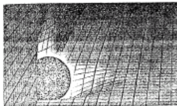
Figura 3.6 Una muestra del espacio tridimensional alabeado que rodea al Sol.
