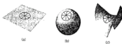
Figura 3.2 Un círculo dibujado sobre una esfera (b) tiene una circunferencia menor que uno que esté dibujado sobre una hoja plana de papel (a), mientras que un círculo dibujado sobre la superficie de una silla de montar (c) tiene una circunferencia mayor, aunque todos estos círculos tengan el mismo radio.
