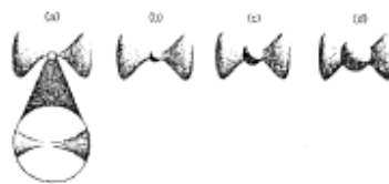
Figura 11.4 Un espacio de Calabi-Yau pinzado se abre rasgándose y crece en él una esfera que se infla alisando su superficie. La esfera original de la Figura 11.3 se ha «ablandado inflándose».
