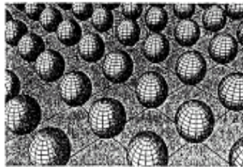
Figura 8.7 Dos dimensiones adicionales arrolladas tomando su forma en la superficie de una esfera.
