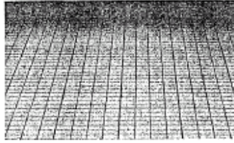
Figura 3.3 Representación esquemática del espacio plano.
