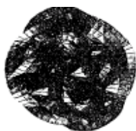
Figura 8.9 Ejemplo de espacio de Calabi-Yau.
