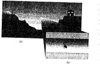
Figura 8.1 (a) Una manguera de riego vista desde una distancia considerable parece un objeto unidimensional. (b) Cuando se amplía, se hace visible una segunda dimensión, una dimensión que tiene forma de círculo y está arrollada en torno a la manguera.
