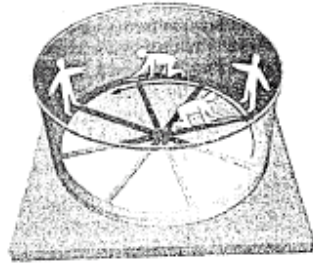
Figura 3.1 La regla de Slim se contrae, porque está colocada en la dirección del movimiento del aparato. Sin embargo, la regla de Jim está colocada a lo largo de una viga radial, perpendicular a la dirección del movimiento del aparato, y en consecuencia su longitud no se contrae.
